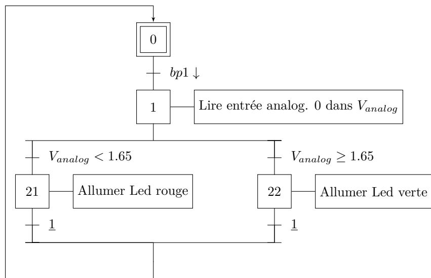
10: Grafcet 10
