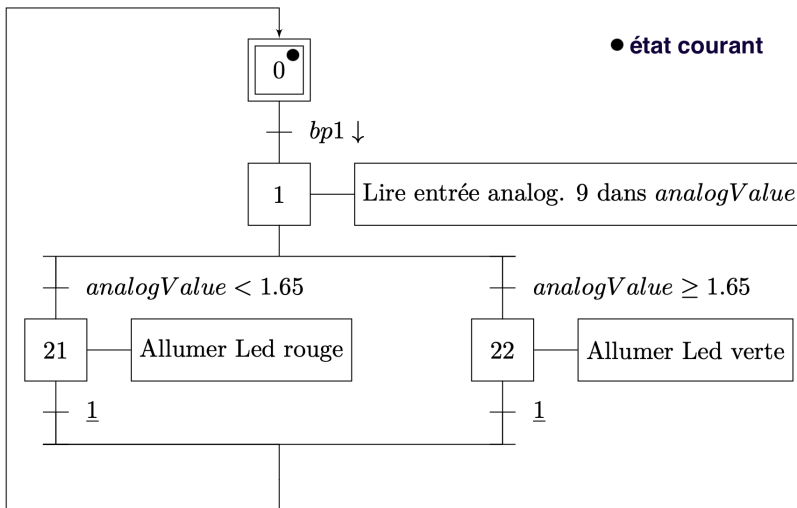
Figure: Entraînement évaluation - GRAFCET 2
