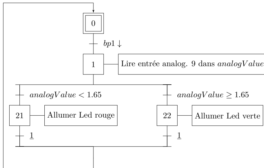
10: Grafcet 10
