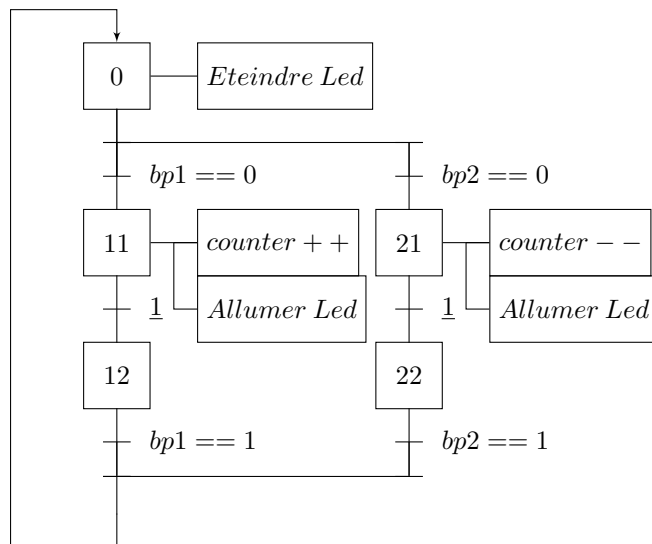
4: Grafcet 4
