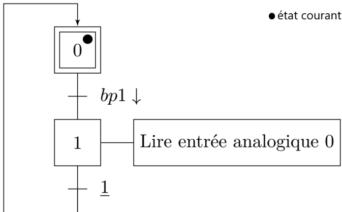
Figure: Entraînement évaluation - GRAFCET 1
