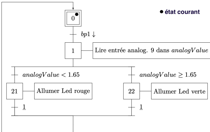
Figure: Entraînement évaluation - GRAFCET 2
