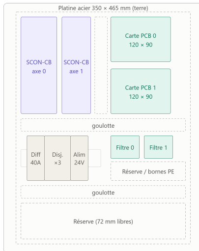
Figure: Schéma d'implantation dans le boîtier
