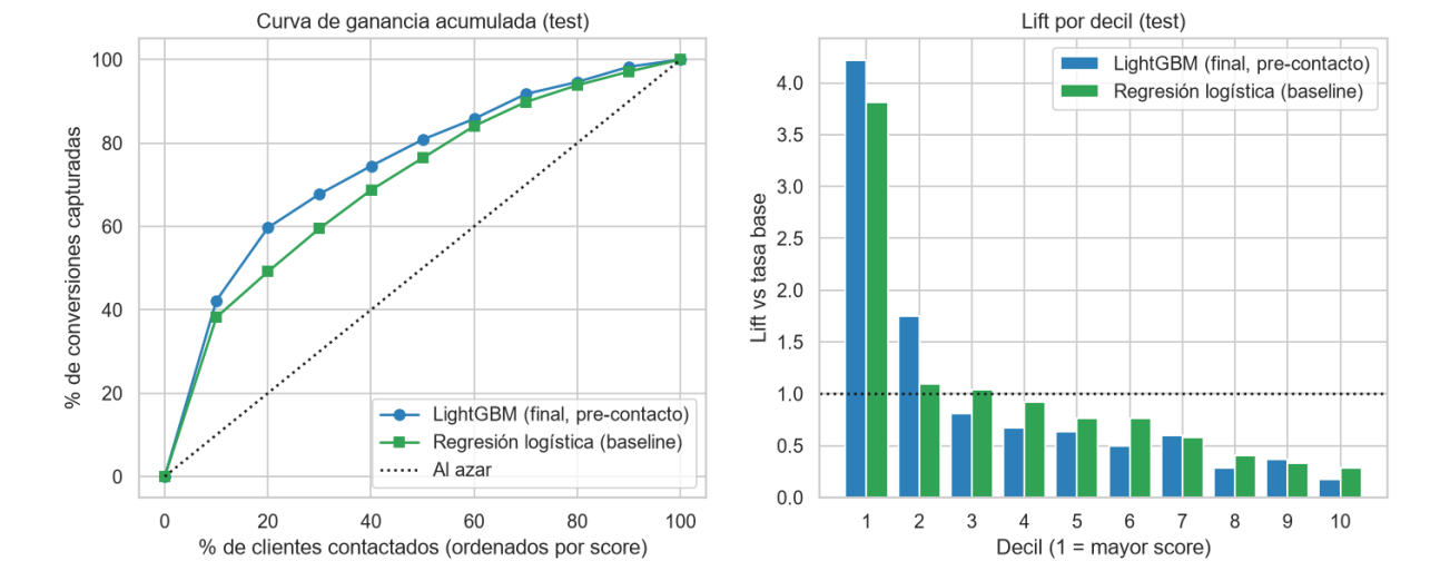
Gain y lift
