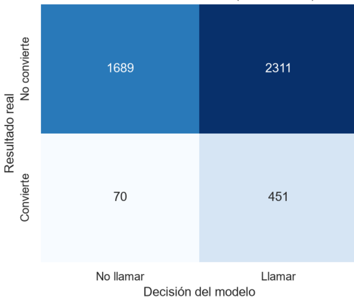
Matriz de confusión en test (umbral 0.050)
