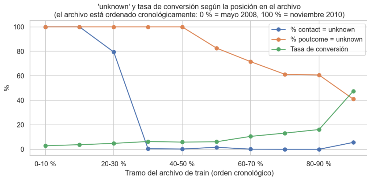
Unknown y conversión a lo largo del archivo
