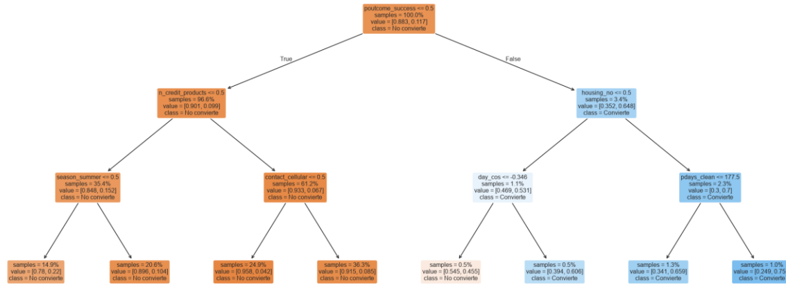
Árbol de reglas
