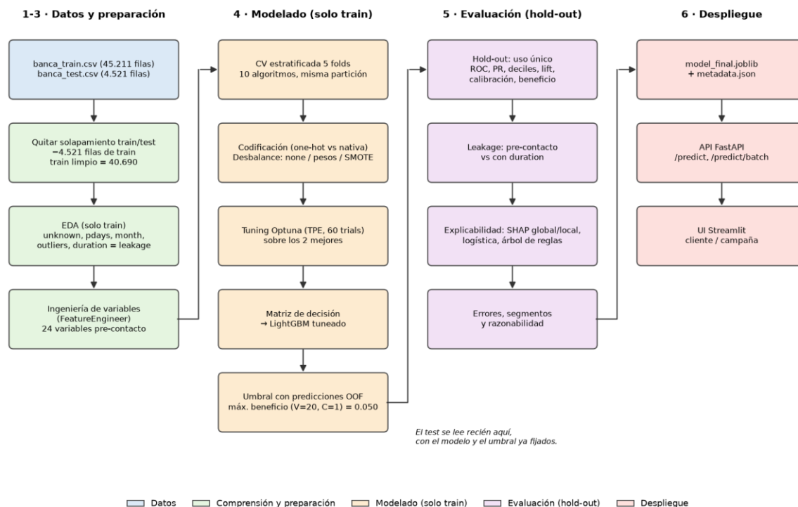
Flujo completo del proyecto (CRISP-DM)
