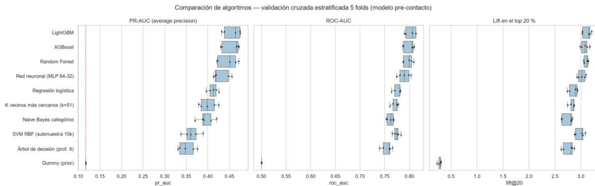
Comparación de algoritmos
