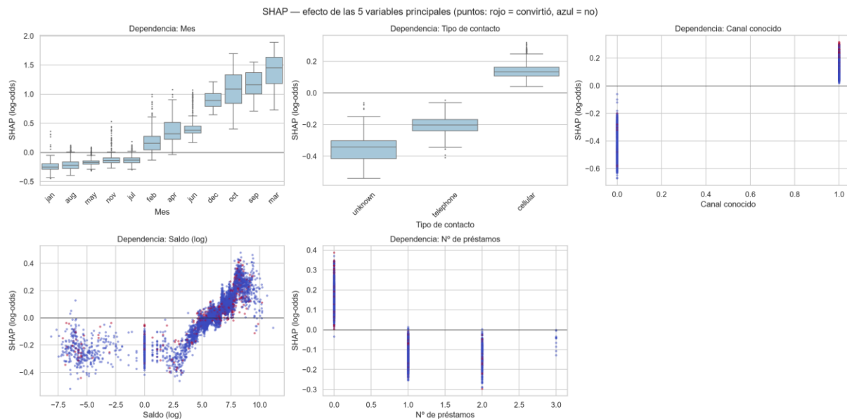
Dependencias SHAP
