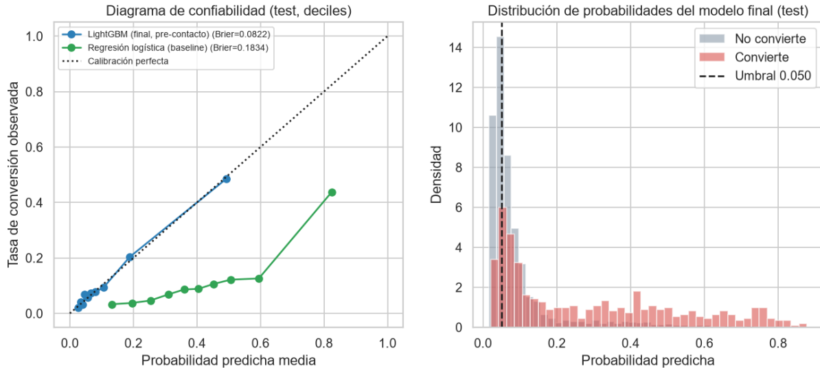
Calibración
