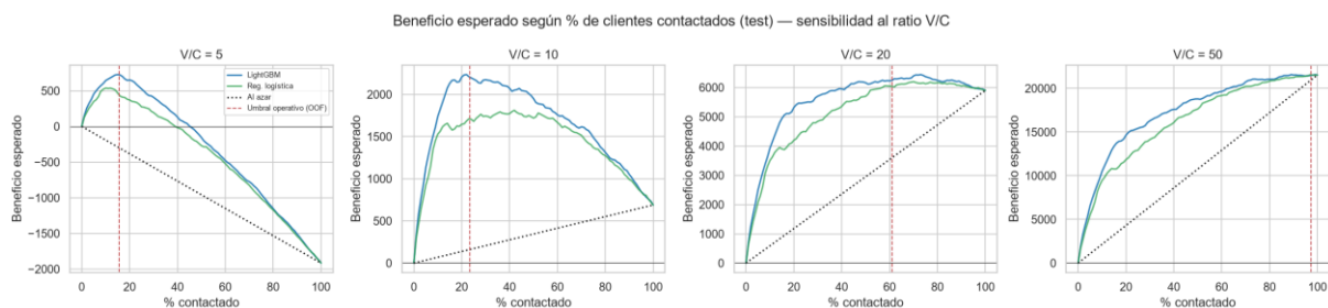
Curvas de beneficio
