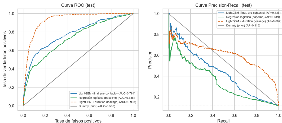
Curvas ROC y PR
