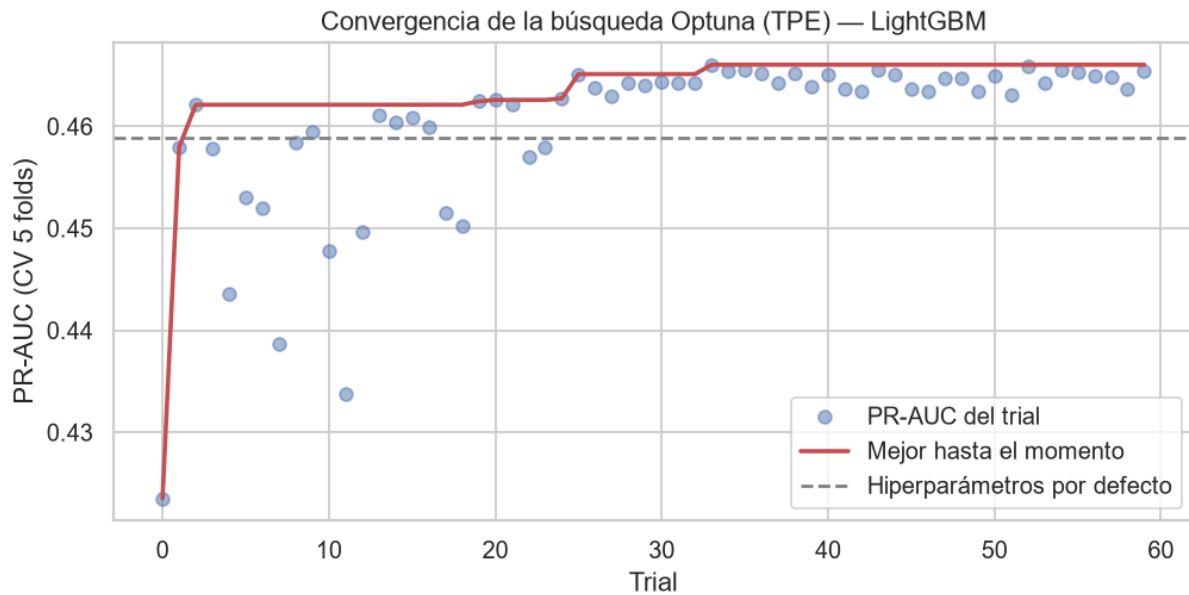
Convergencia Optuna LightGBM
