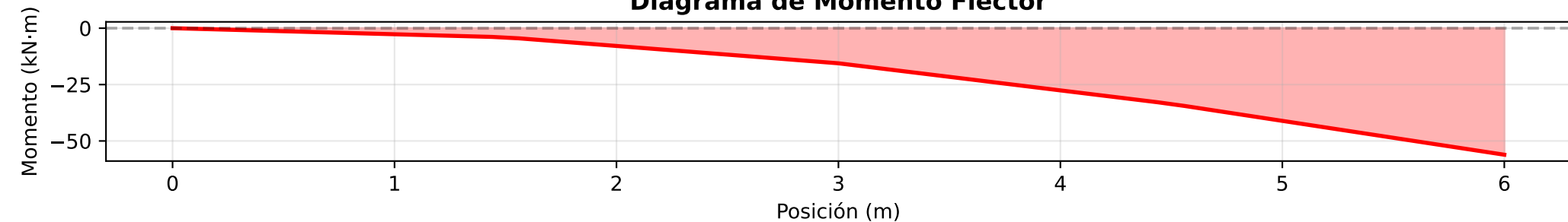
Diagrama de Momento Flector
