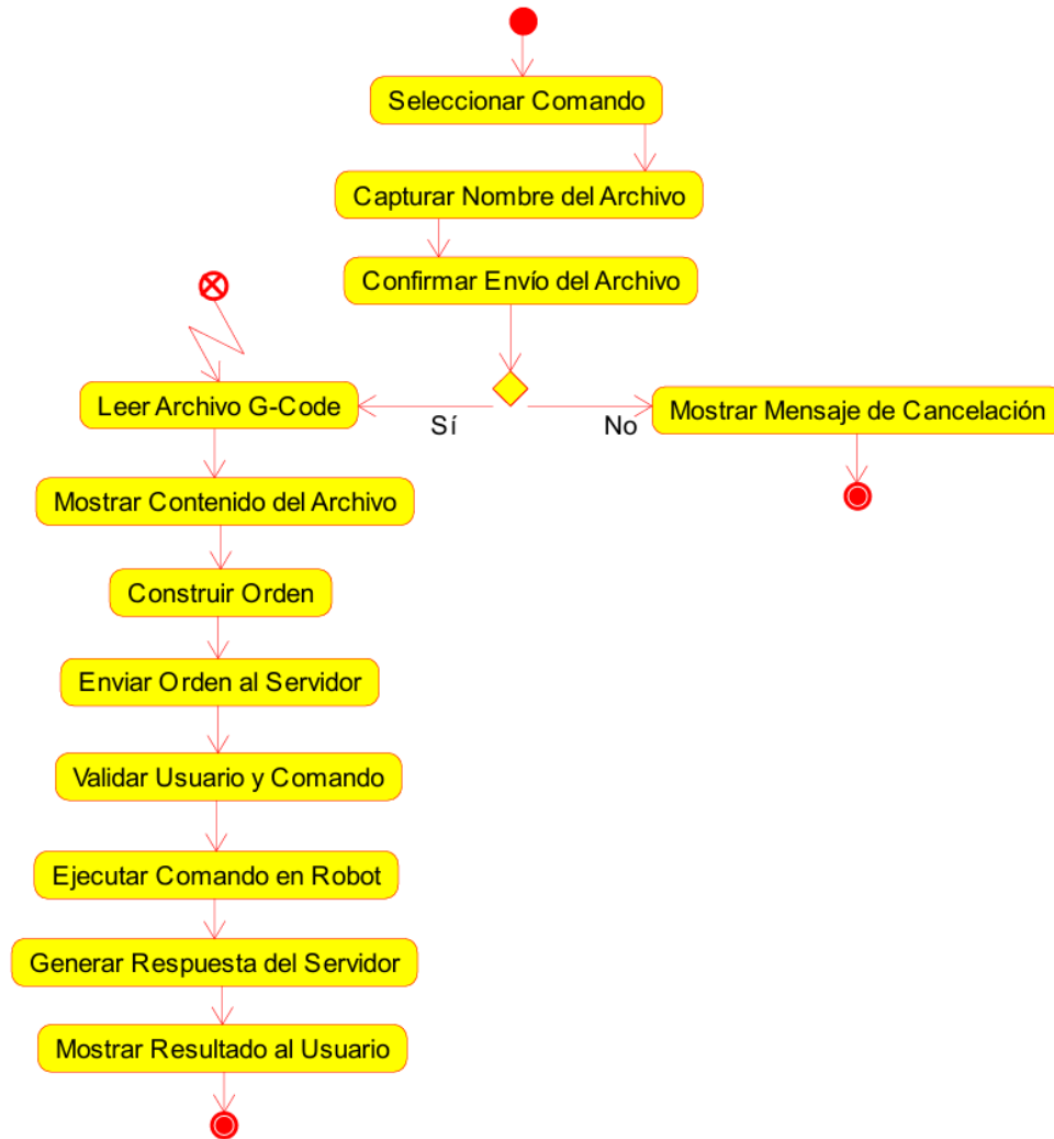
Figure 6: Diagrama de actividad: Ejecución de Comando G-Code
