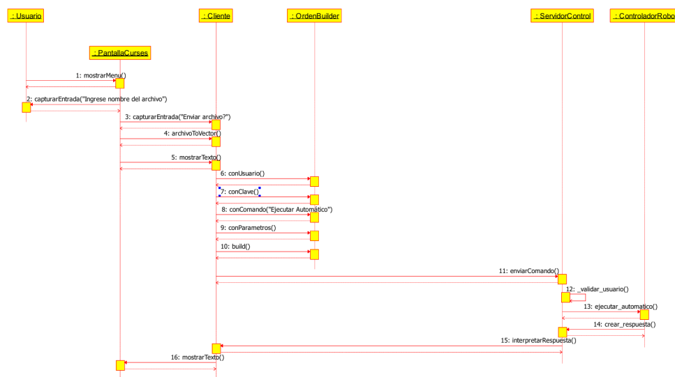
Figure 4: Diagrama de secuencia: Ejecutar Comando con Archivo G-Code
