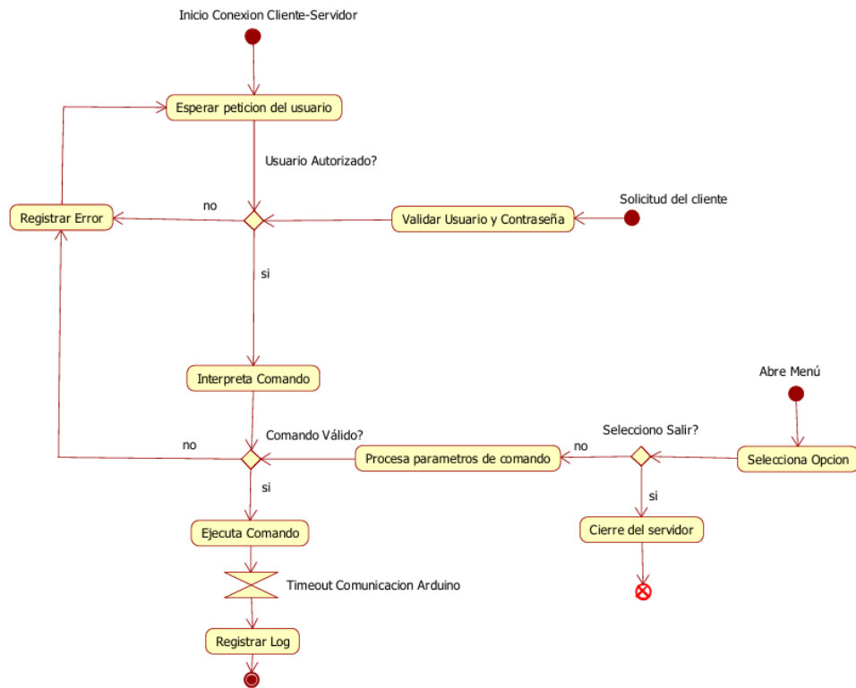
Figure 5: Diagrama de actividad general
