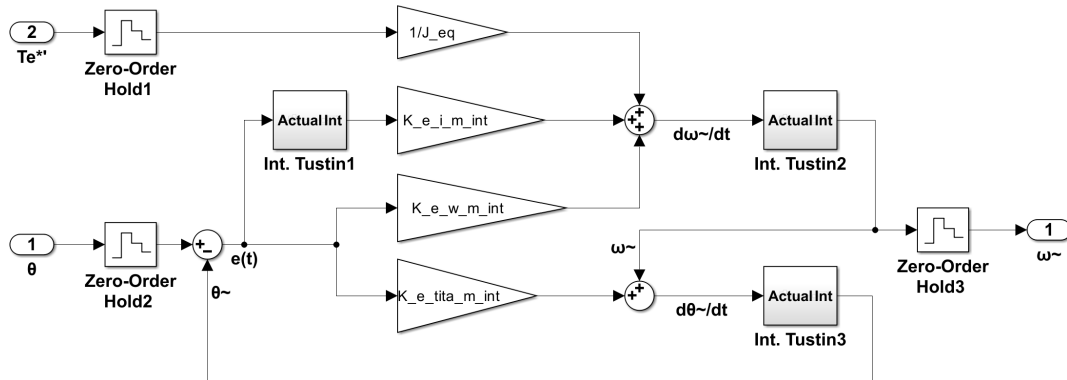
Fig. 63. Diagrama de bloques del observador discretizado. Incorporación de ZOH y reemplazo de integradores continuos por integradores de Tustin.
