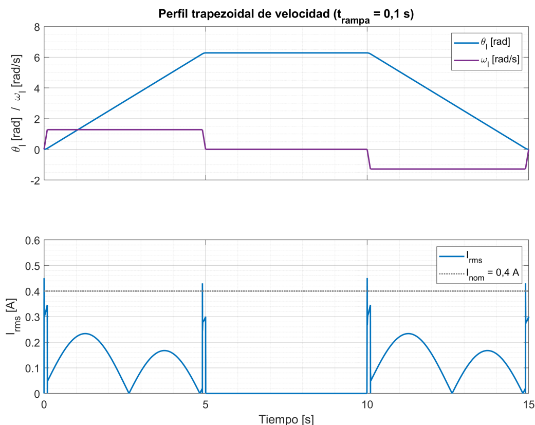
Fig. 53. En este caso, con un tiempo de rampa de t = 0,1 \text{ s} , puede verse que la corriente pico apenas supera los 0,4 A.
