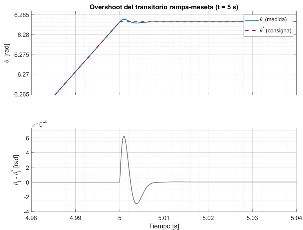
Fig. 45. Overshoot del transitorio rampa-meseta de la posición de la articulación
