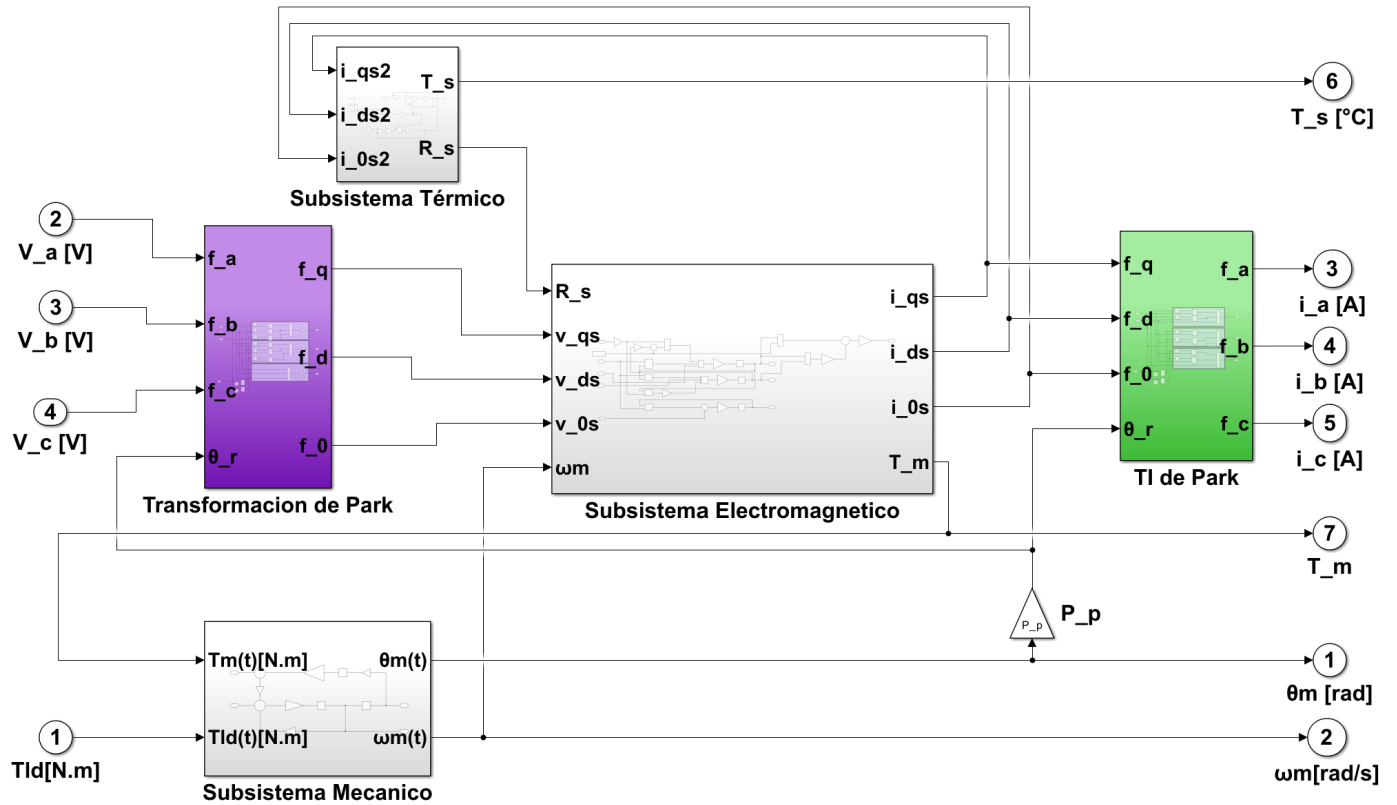
Fig. 3. Diagrama de bloques del modelo del accionamiento implementado en Simulink. Las Transformaciones de Park directa e inversa vinculan el marco de fase abc con el marco rotórico qd0 , y se muestra la interconexión de los subsistemas electromagnético, mecánico y térmico.
