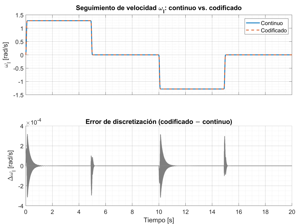
Fig. 73. Comparación de seguimiento de consigna de velocidad del modelo continuo vs el codificado discreto.
