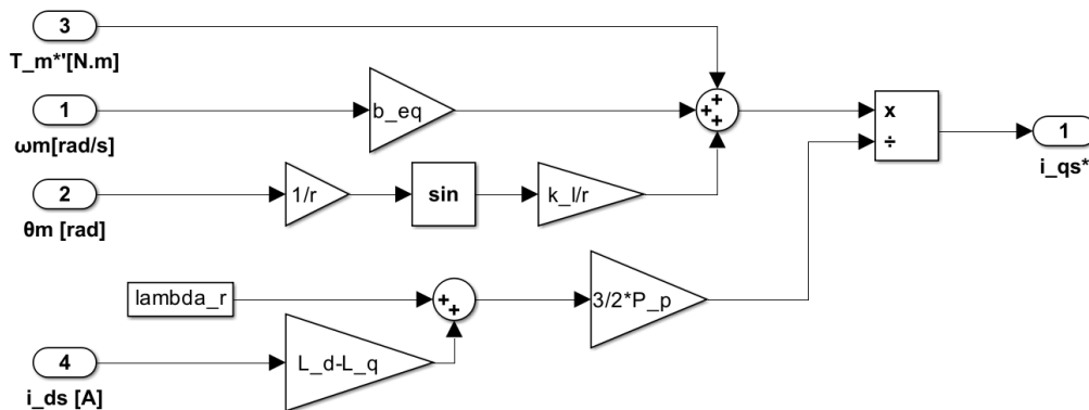
Fig. 38. Diagrama de bloques del modulador de torque implementado.
