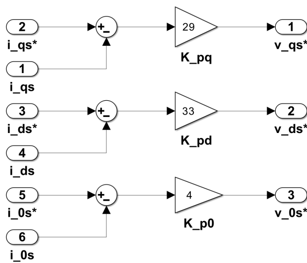
Fig. 36. Lazos de control de corriente i_{qd0s}^r con acción proporcional, ubicando los polos del lazo interno en p_i = -5000 rad/s.
