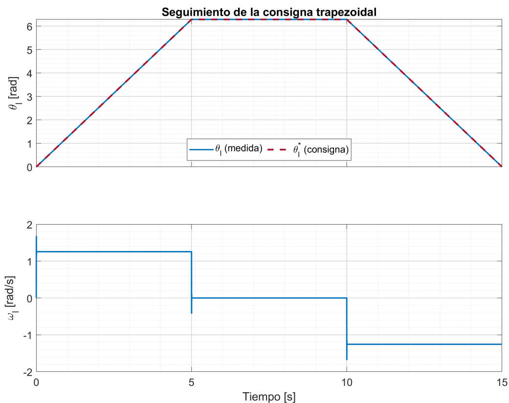
Fig. 44. Posición y velocidad de la articulación en función del tiempo siguiendo la consigna trapezoidal propuesta
