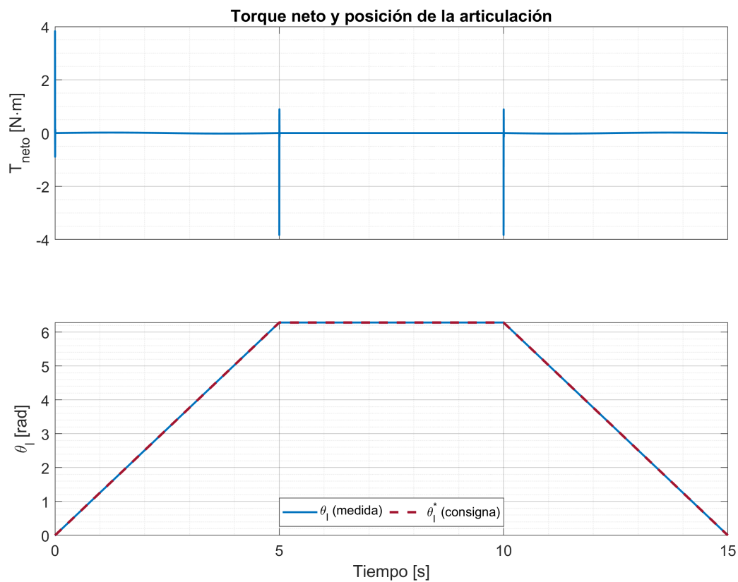
Fig. 46. Torque neto aplicado por la articulación para seguir la consigna de posición.
