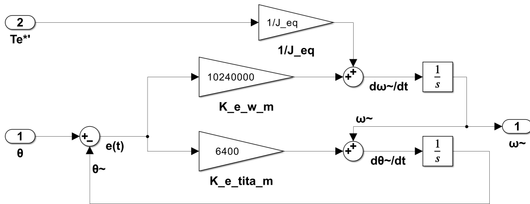
Fig. 43. Diagrama de bloques del observador de estados reducido
