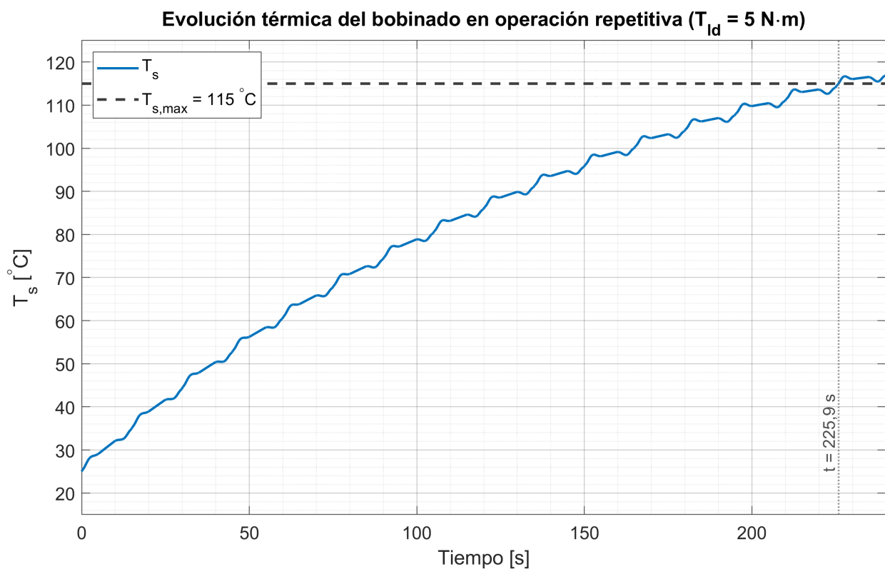
Fig. 58. Evolución de la temperatura del bobinado T_s^\circ(t) bajo operación repetitiva, considerando T_{amb}^\circ = 25^\circ\text{C} , T_{ld} = 5 \text{ Nm} y la consigna trapezoidal de posición utilizada en el trabajo. Se observa que la temperatura supera el límite admisible T_{s,max}^\circ = 115^\circ\text{C} a los 225,9 s.
