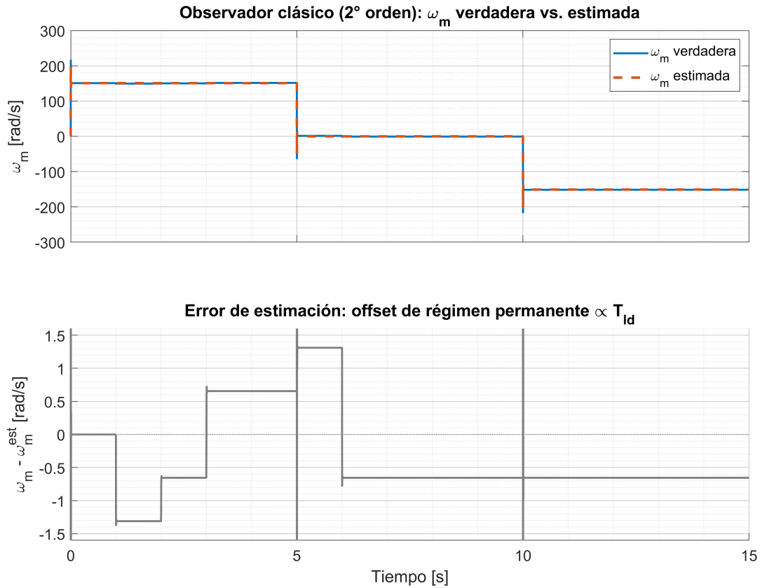
Fig. 55. Error de offset observado con el observador mecánico de segundo orden sin acción integral, ante perturbaciones de carga cuasi-estacionarias.
