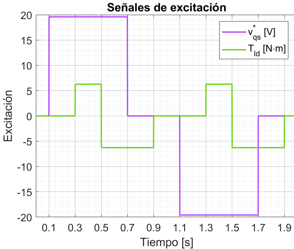
Fig. 14. Señales de excitación: consigna de tensión v_{qs}^{r*}(t) y torque de carga T_{ld}(t) .
