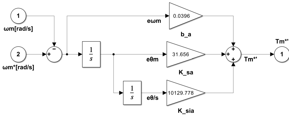
Fig. 40. Implementación en Simulink del controlador PID externo de movimiento. La entrada es el error de velocidad e_\omega = \omega_m^* - \omega_m ; su integral reconstruye el error de posición e_{\theta m} y una segunda integración provee la acción integral. Las tres ramas ponderadas por b_a , K_{sa} y K_{sia} se suman para entregar la consigna de torque T_m^{*l} , realizando la ley (97).
