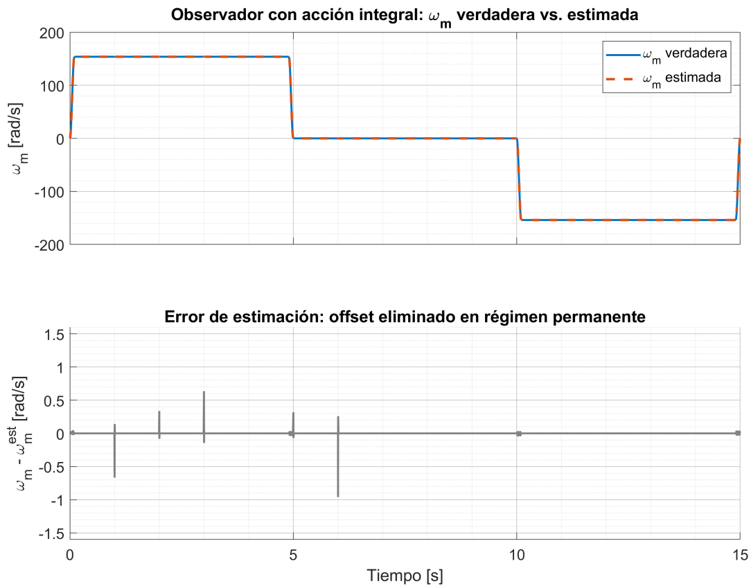
Fig. 57. Respuesta del observador aumentado con acción integral. Se observa la desaparición del error de offset en régimen permanente.
