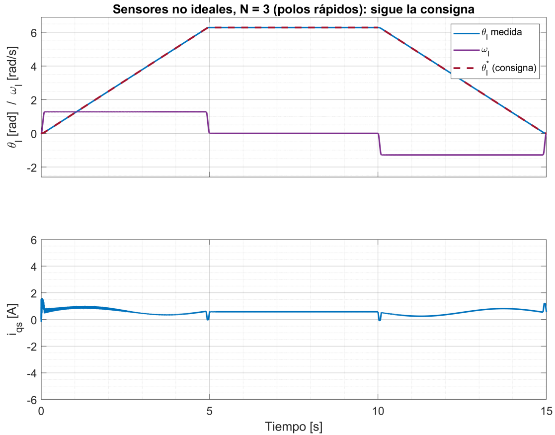
Fig. 60. Arriba: posición y velocidad; abajo: corriente en eje de cuadratura. Puede verse que el accionamiento ya sigue con éxito la consigna solicitada, sin oscilaciones producidas por los retardos de los sensores. ( T_{ld} = 5 [Nm])
