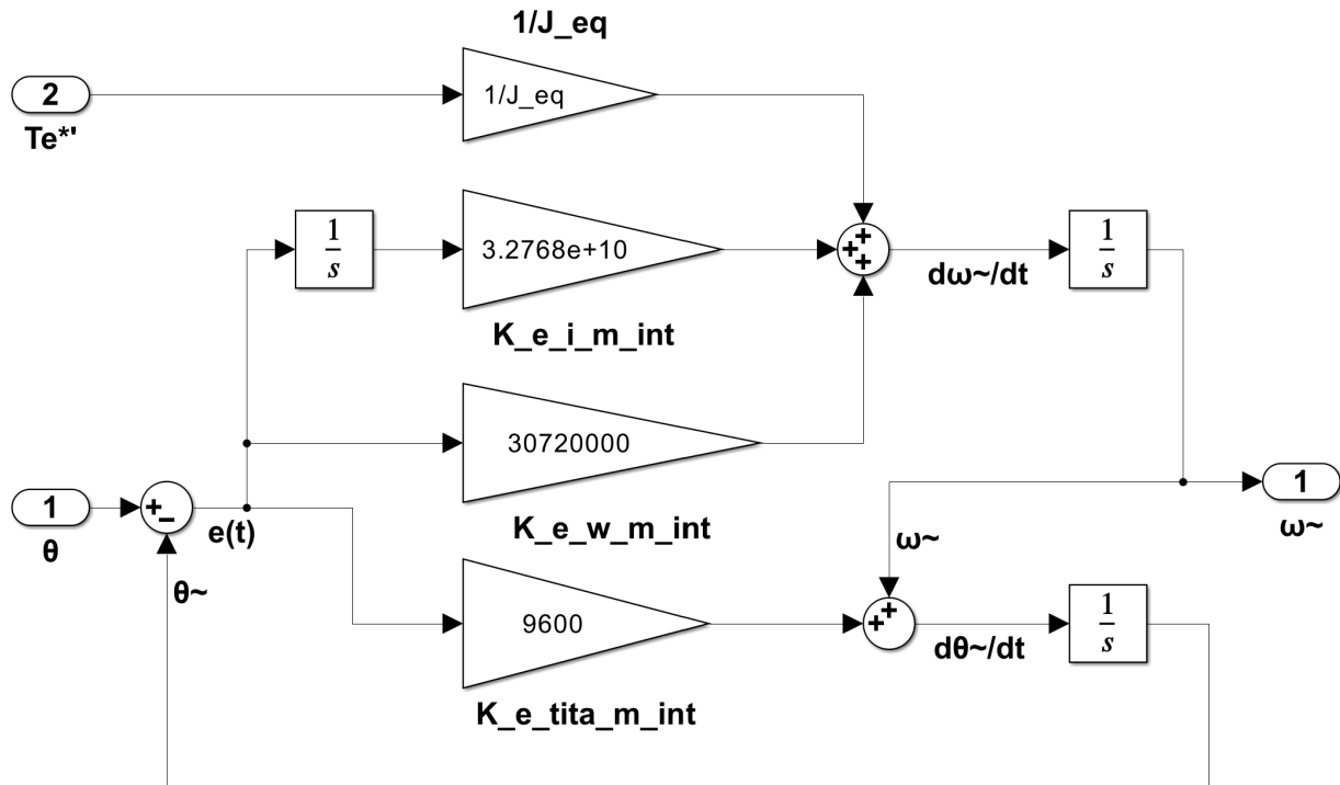
Fig. 56. Diagrama de bloques del observador mecánico aumentado con acción integral implementado en Simulink. El error de posición e_\theta(t) = \theta_m(t) - \hat{\theta}_m(t) alimenta tanto las ramas proporcionales como la rama integral, cuya salida corrige la dinámica de \hat{\omega}_m(t) para eliminar el error estacionario de estimación.
