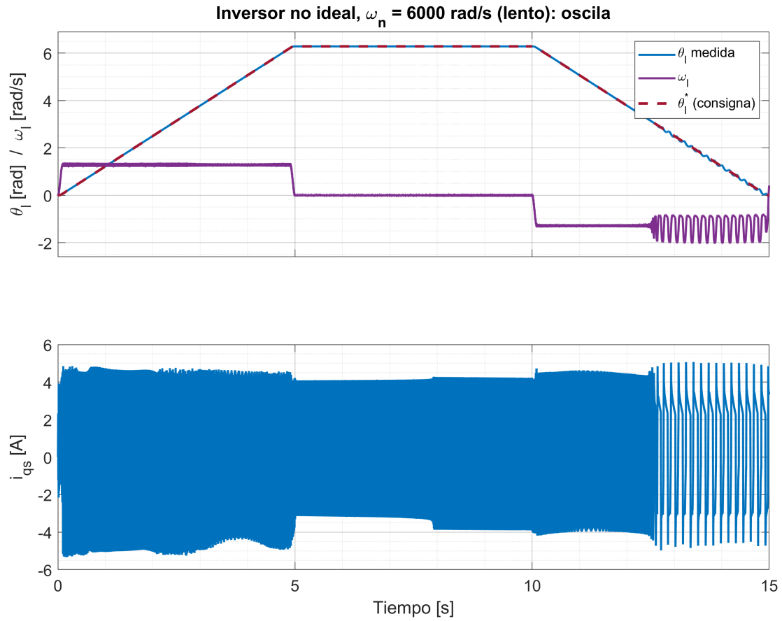
Fig. 61. Arriba: posición y velocidad; abajo: corriente en eje de cuadratura. Puede verse que el inversor no es lo suficientemente rápido. ( T_{ld} = 5 [Nm], \omega_n = 6000 [rad/s])
