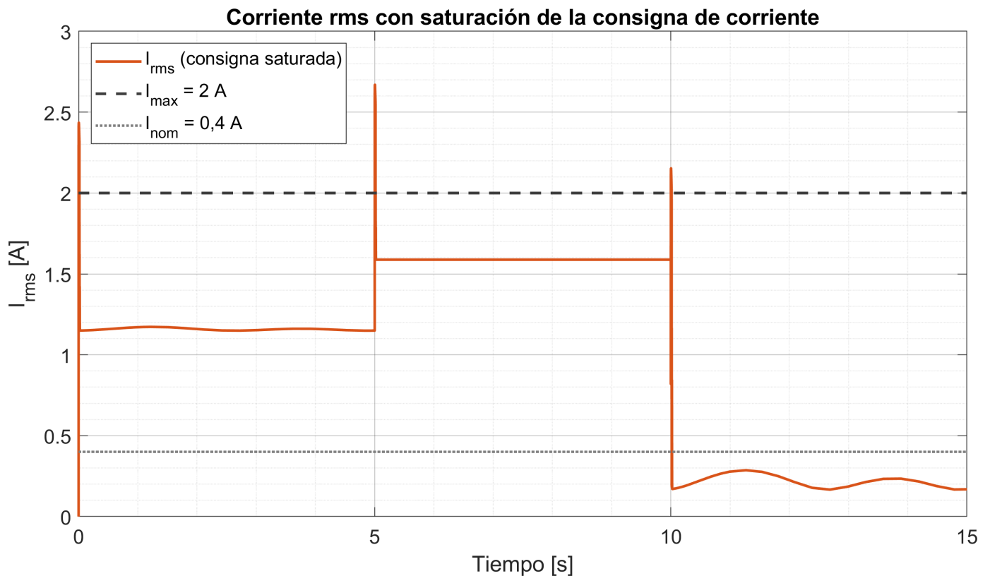
Fig. 52. Puede verse que, aun con saturación en la consigna de corriente, el accionamiento no puede cumplir la consigna sin superar sus especificaciones.
