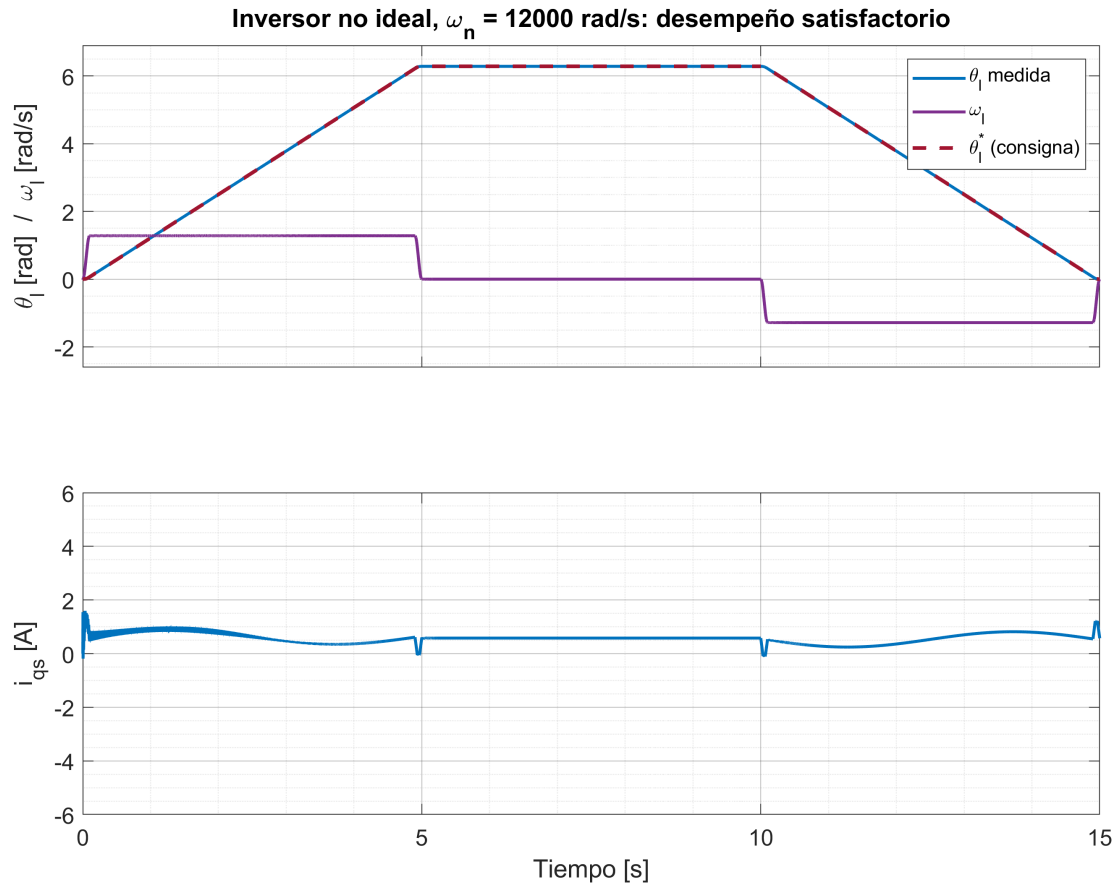
Fig. 62. Arriba: posición y velocidad; abajo: corriente en eje de cuadratura. Finalmente se consigue un desempeño satisfactorio y, al mismo tiempo, el cumplimiento de las demás condiciones de operación. ( T_{ld} = 5 [Nm], \omega_n = 12000 [rad/s])
