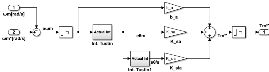
Fig. 64. Diagrama de bloques del controlador de posición discretizado. Incorporación de ZOH y reemplazo de integradores continuos por integradores de Tustin.
