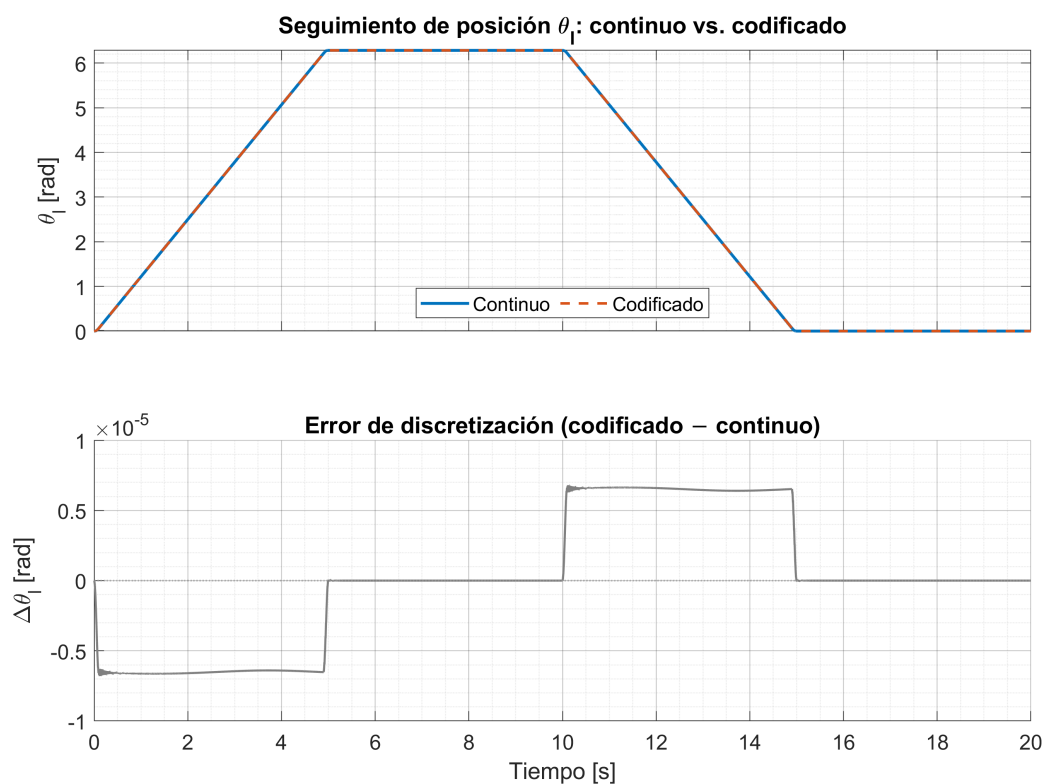
Fig. 72. Comparación de seguimiento de consigna de posición del modelo continuo vs el codificado discreto.
