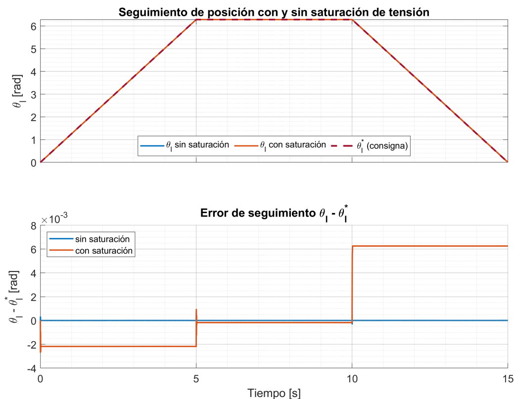
Fig. 51. Seguimiento de posición con y sin saturación de tensión del inversor (39,19 V). El seguimiento es prácticamente idéntico en ambos casos; el error de posición se mantiene en el orden de 10^{-3} rad.
