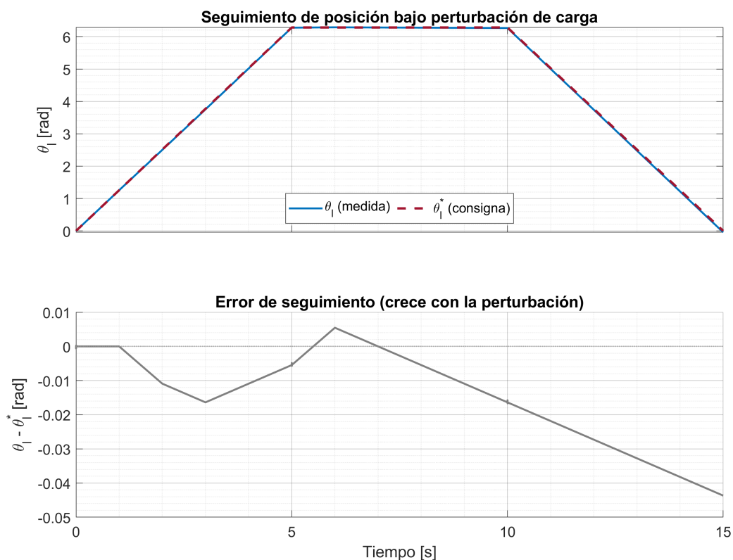
Fig. 48. Influencia del torque de perturbación en el seguimiento de la consigna de posición y el error creciente.
