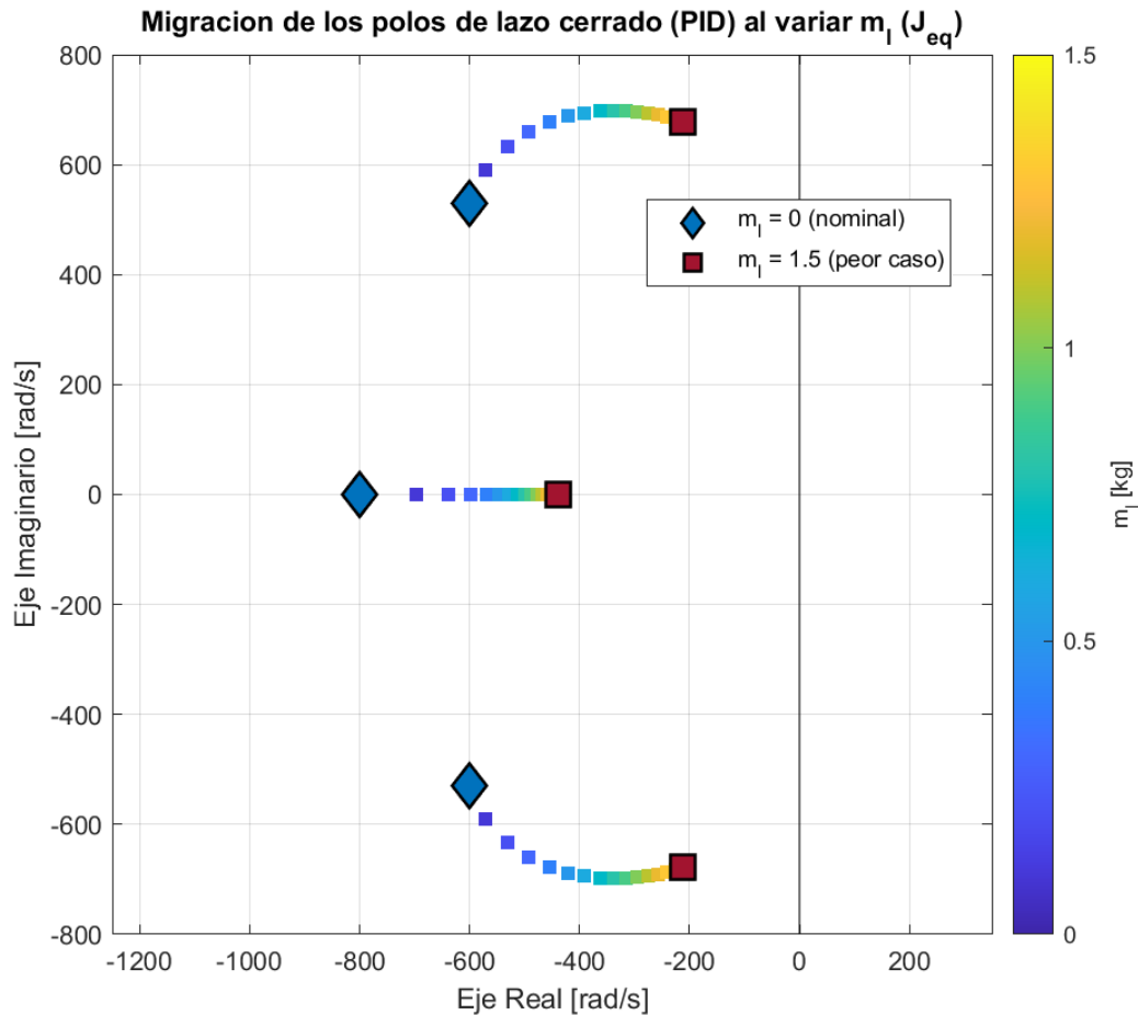
Fig. 42. Migración de los polos de lazo cerrado del PID al variar m_l de 0 a 1,5 kg con ganancias fijas (cuadrados sólidos, colorbar en m_l ). El nominal ( m_l = 0 ) se marca con rombo sólido y el peor caso ( m_l = 1,5 ) con cuadrado sólido.
