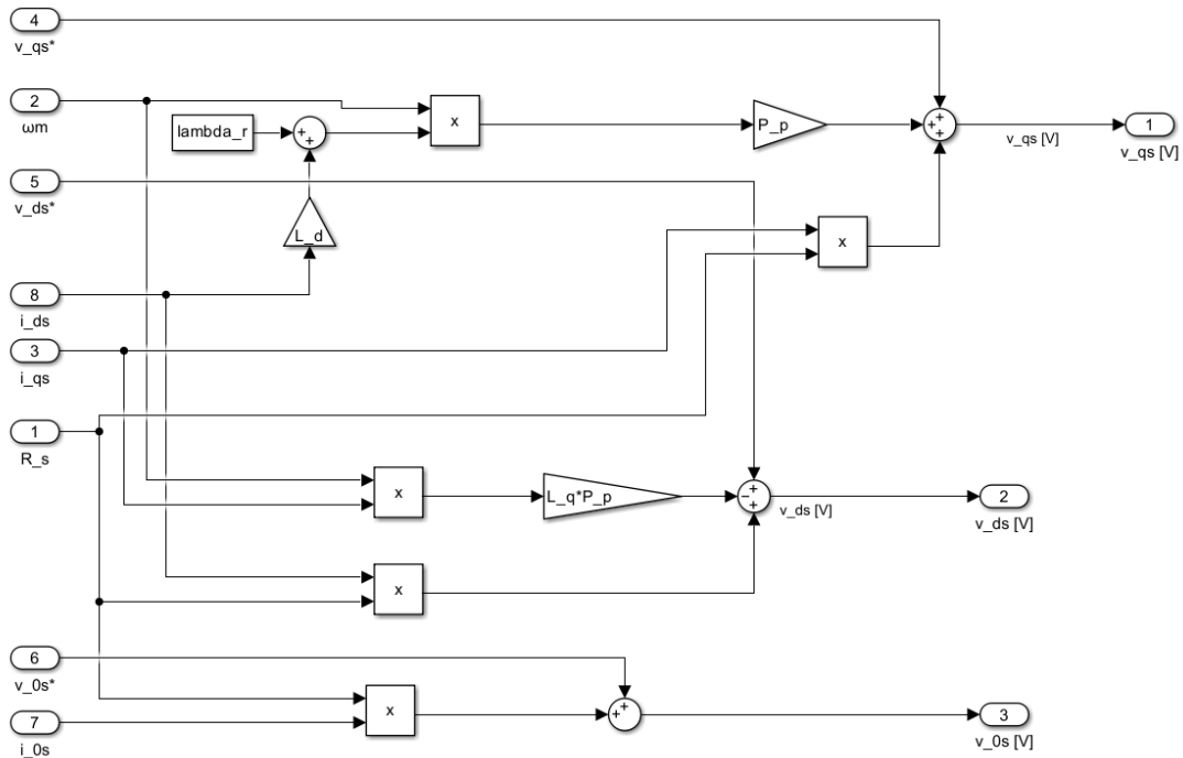
Fig. 32. Implementación en Simulink del desacoplamiento de las retroalimentaciones físicas naturales: las tensiones de referencia v_{qd0s}^{r*} cancelan las caídas resistivas R_s(T_s^\circ) i , la fuerza contraelectromotriz y los acoplamientos cruzados entre los ejes q y d .
