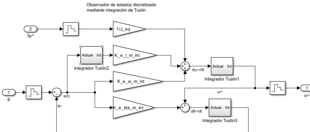
Fig. 62. Diagrama de bloques del observador discretizado. Incorporación de ZOH y reemplazo de integradores continuos por integradores de Tustin.
