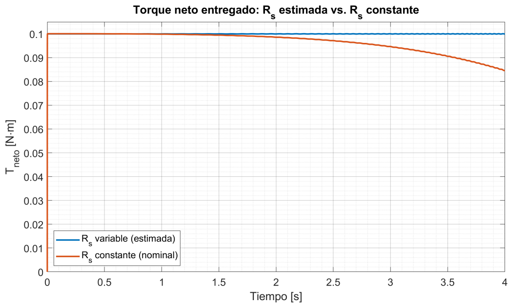
Fig. 34. Evolución temporal del torque neto ( T_{\text{neto}} ) en [N.m]. Se contrasta el comportamiento con resistencia estática constante ( R_s Cte., línea naranja) y con resistencia estática variable ( R_s Variable, línea azul).
