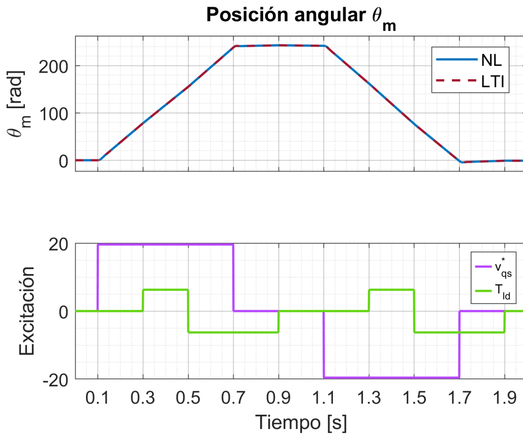
Fig. 16. Posición angular \theta_m(t) : comparación NL (azul) vs LTI aumentado (rojo). Panel inferior: señales de excitación (torque de carga T_l y consigna v_{qs}^* ).
