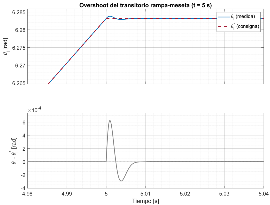
Fig. 44. Overshoot del transitorio rampa-meseta de la posición de la articulación
