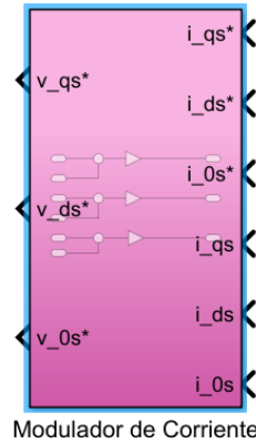
Fig. 37. Subsistema del modulador (lazo proporcional) de corrientes.
