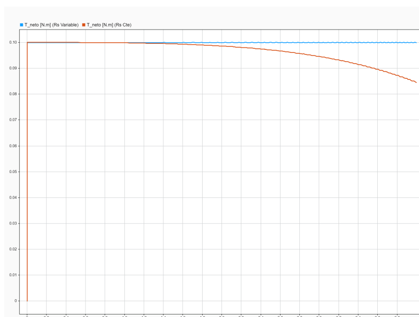
Fig. 36. Evolución temporal del torque neto ( T_{\text{neto}} ) en [N.m]. Se contrasta el comportamiento con resistencia estática constante (RS Cte., línea roja) y con resistencia estática variable (RS Variable, línea azul).
