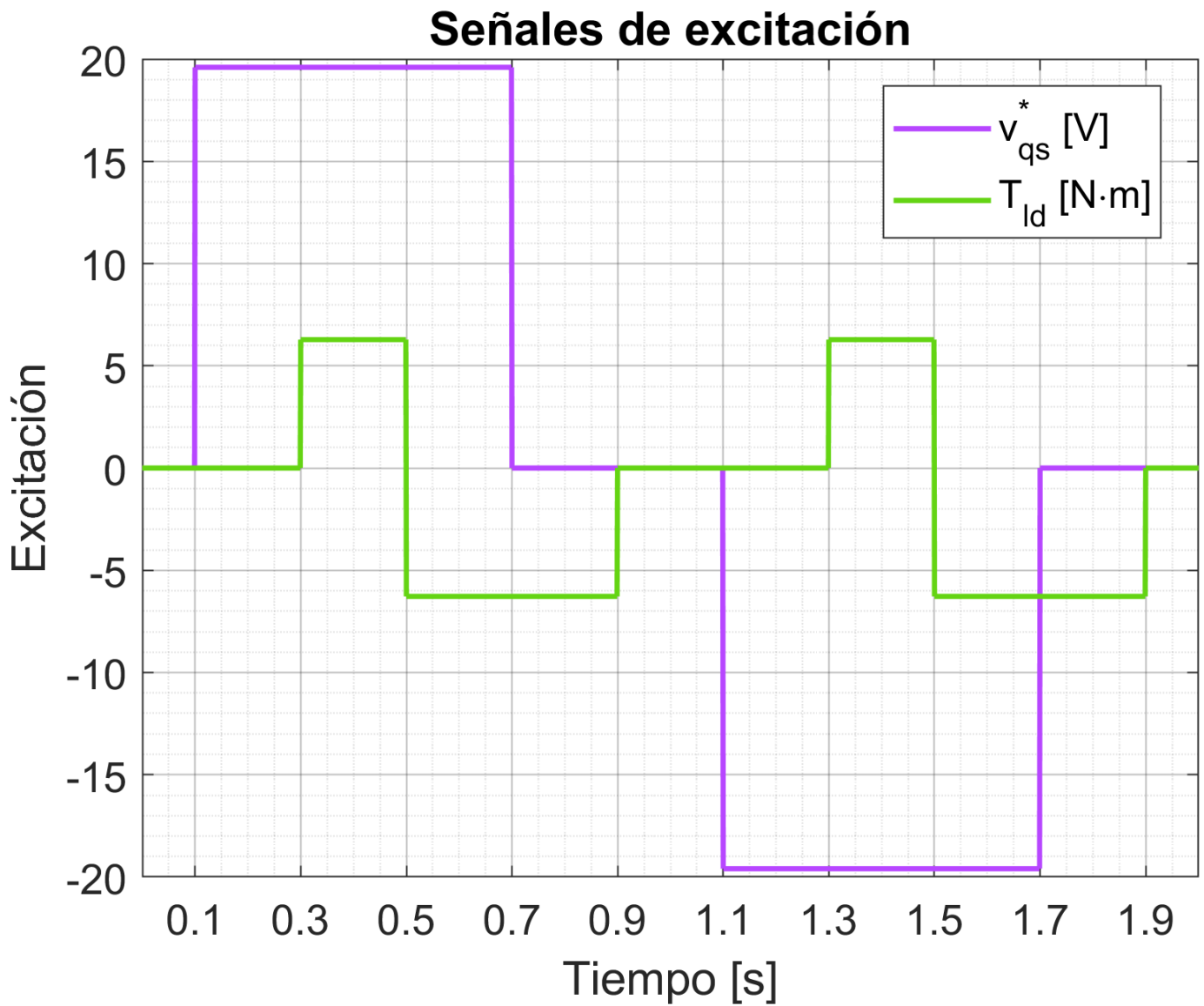
Fig. 16. Señales de excitación: consigna de tensión v_{qs}^{r*}(t) y torque de carga T_{ld}(t) .
