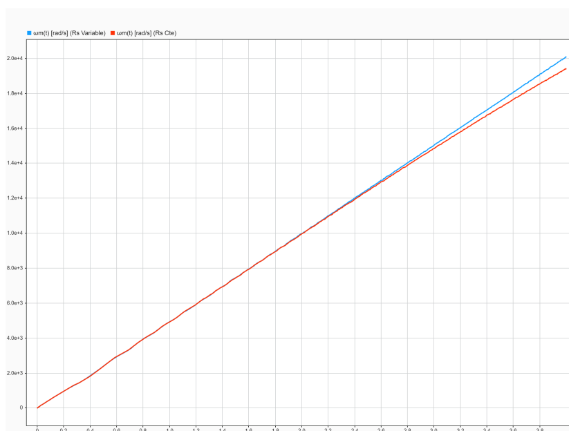
Fig. 37. Comportamiento de la velocidad angular mecánica ( \omega_m(t) ) en [rad/s] en función del tiempo. Se comparan las respuestas con resistencia estática constante (RS Cte., línea roja) y con resistencia estática variable (RS Variable, línea azul).
