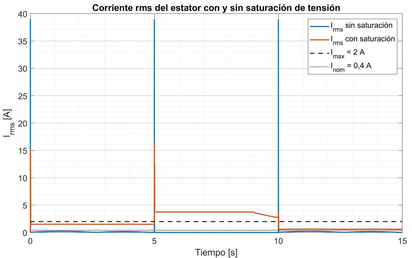
Fig. 51. Comparación de la corriente rms del estator con y sin limitación de la tensión del inversor.
