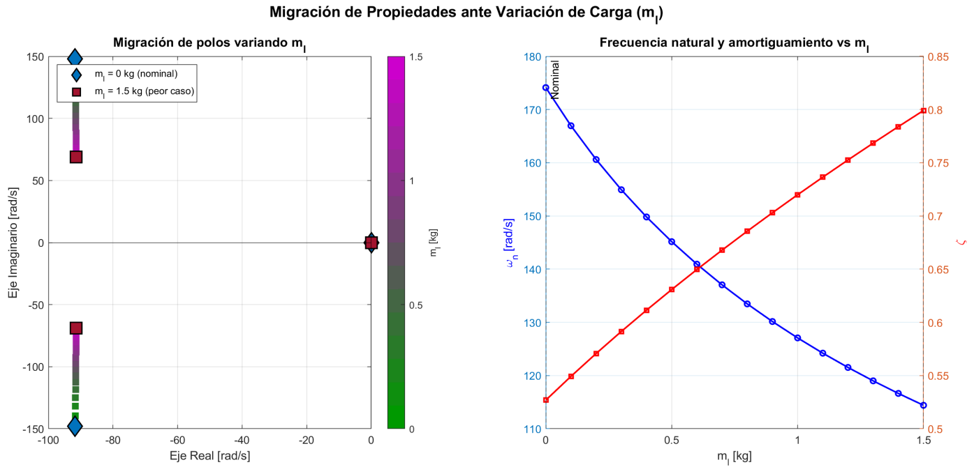
Fig. 14. Migración de polos ante variación de masa de carga m_l (izquierda) y variación de \omega_n y \zeta (derecha).
