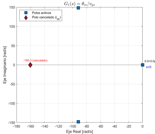
Mapa de Polos y Ceros a Lazo Abierto (Modelo LTI Aumentado)
