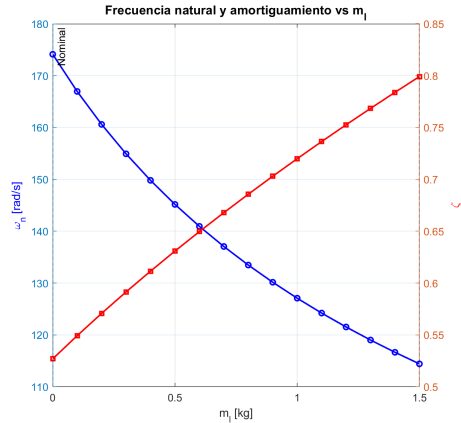
Migración de Propiedades ante Variación de Carga ( m_l )
