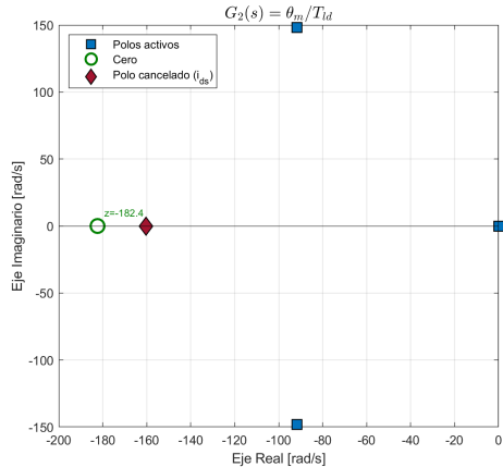
Mapa de Polos y Ceros a Lazo Abierto (Modelo LTI Aumentado)
