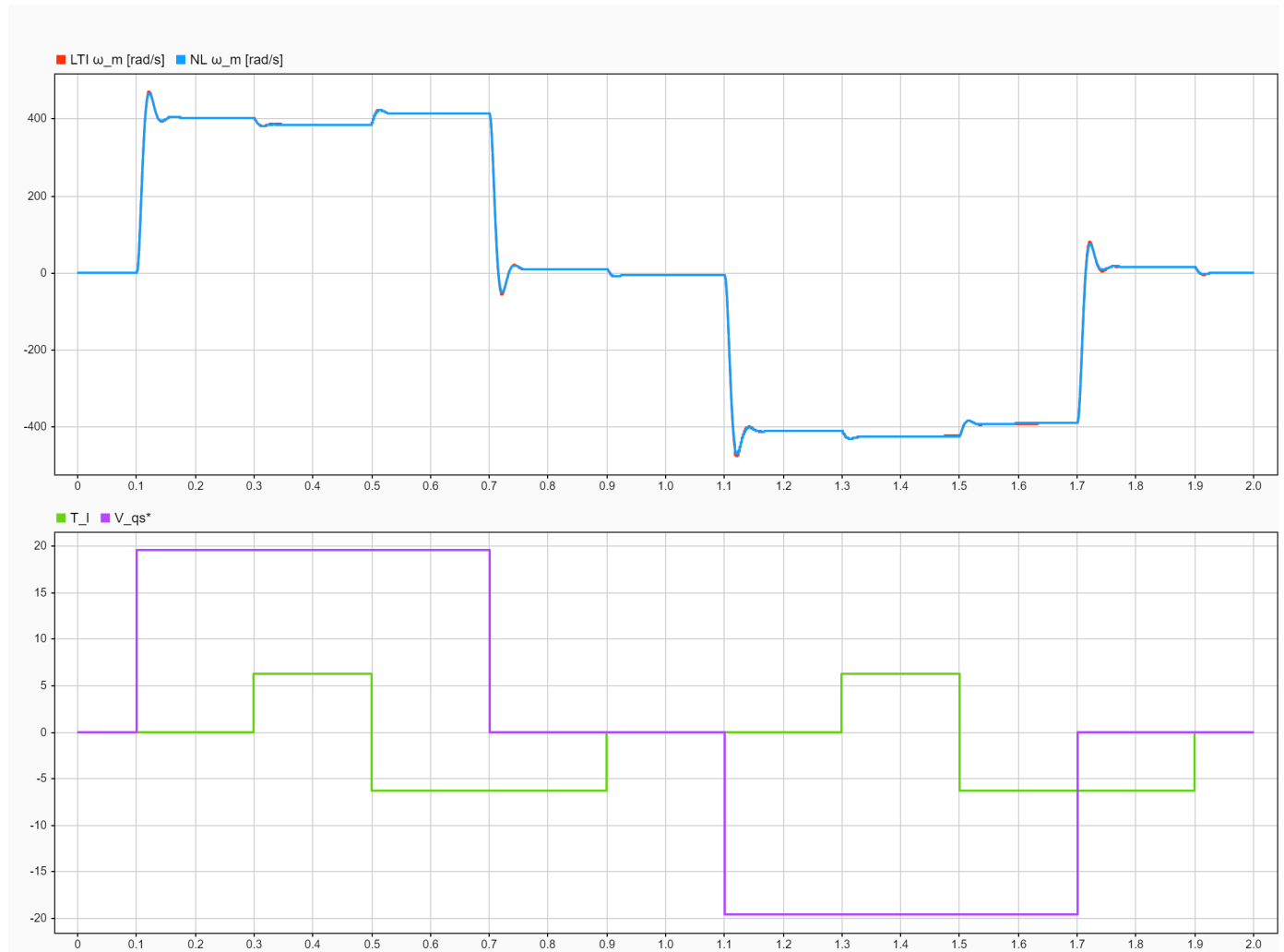
Fig. 18. Velocidad angular \omega_m(t) : comparación NL (azul) vs LTI aumentado (rojo). Panel inferior: señales de excitación ( T_l y v_{qs}^* ).
