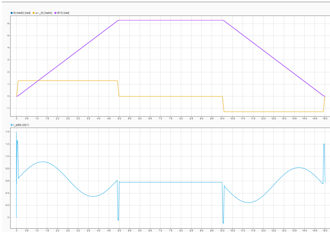
Fig. 59. Arriba: posición y velocidad; abajo: corriente en eje de cuadratura. Puede verse que el accionamiento ya sigue con éxito la consigna solicitada, sin oscilaciones producidas por los retardos de los sensores. ( T_{ld} = 5 [Nm])
