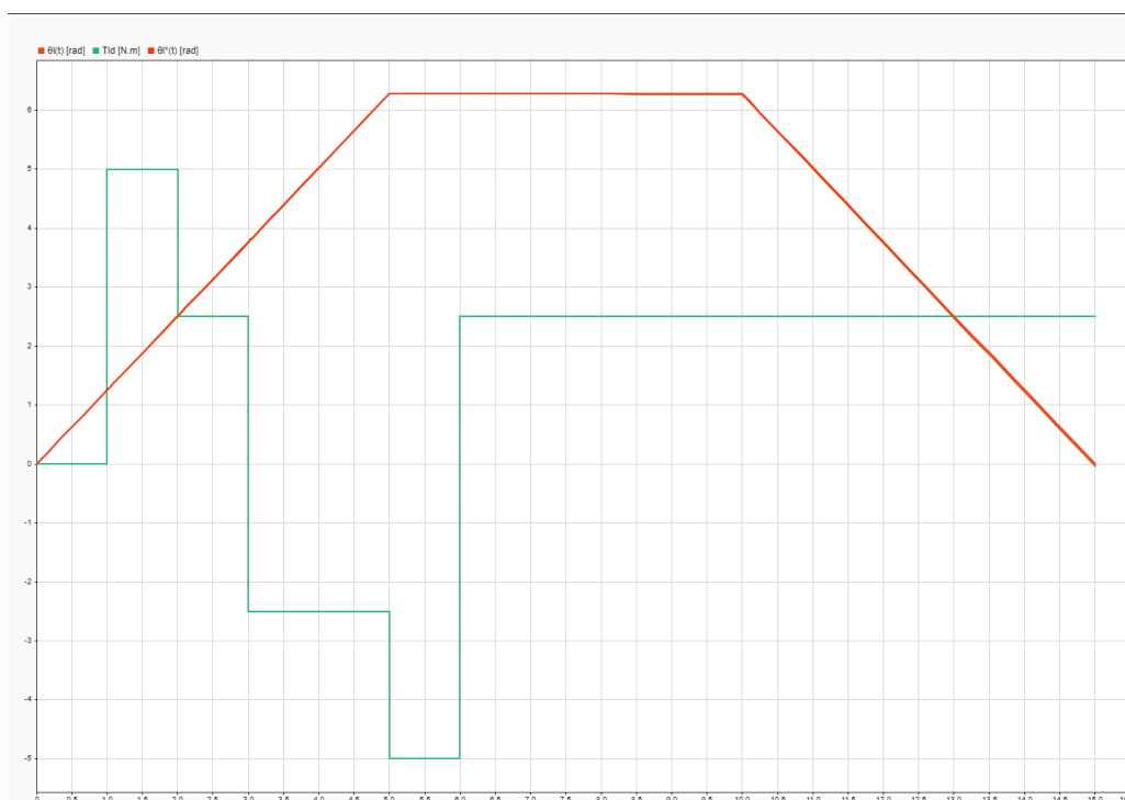
Fig. 47. Perturbación, consigna y posición medida. Puede verse claramente el error que aumenta con el tiempo.
