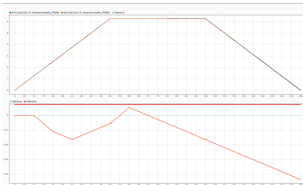
Fig. 46. Influencia del torque de perturbación en el seguimiento de la consigna de posición y el error creciente.
