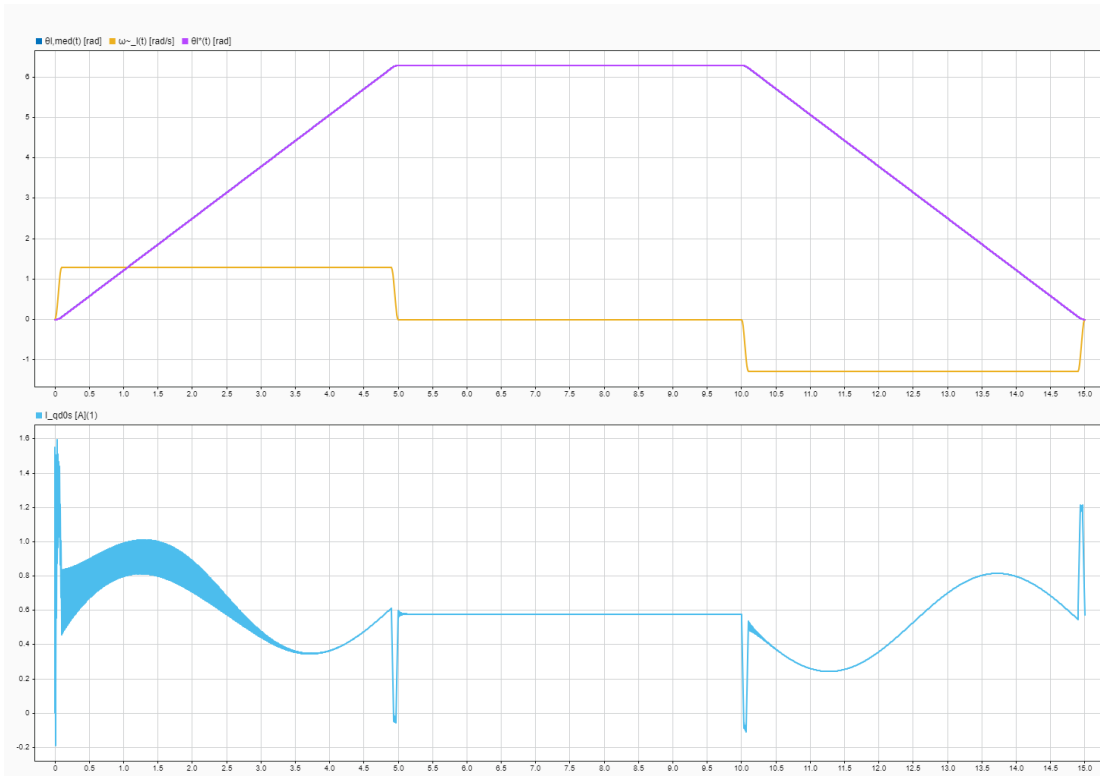
Fig. 61. Arriba: posición y velocidad; abajo: corriente en eje de cuadratura. Finalmente se consigue un desempeño satisfactorio y, al mismo tiempo, el cumplimiento de las demás condiciones de operación. ( T_{ld} = 5 [Nm], \omega_n = 12000 [rad/s])
