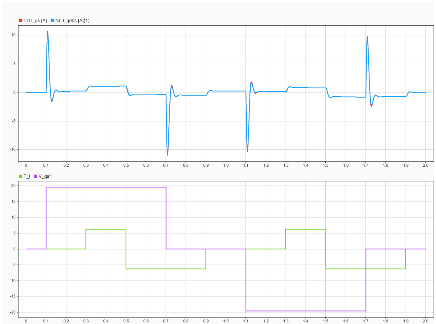
Fig. 20. Corriente de eje q , i_{qs}^r(t) : comparación NL (azul) vs LTI aumentado (rojo). Panel inferior: señales de excitación ( T_l y v_{qs}^{r*} ).
