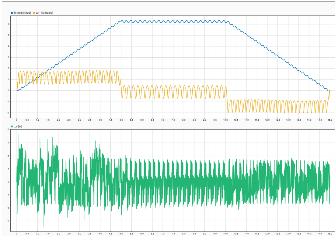
Fig. 58. Arriba: posición y velocidad; abajo: corriente en eje de cuadratura. Puede verse el efecto del modelo en SS de los sensores, con el cual el sistema no puede seguir la consigna de posición. ( T_{id} = 5 [Nm])
