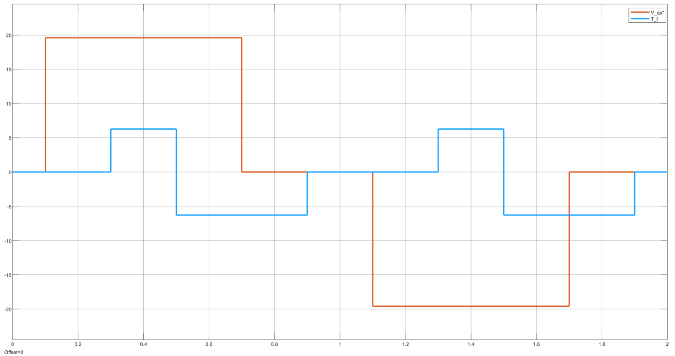
Fig. 14. Señales de excitación: consigna de tensión v_{qs}^{r*}(t) y torque de carga T_{ld}(t) .
