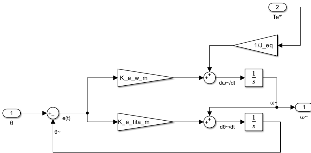
Fig. 41. Diagrama de bloques del observador de estados reducido
