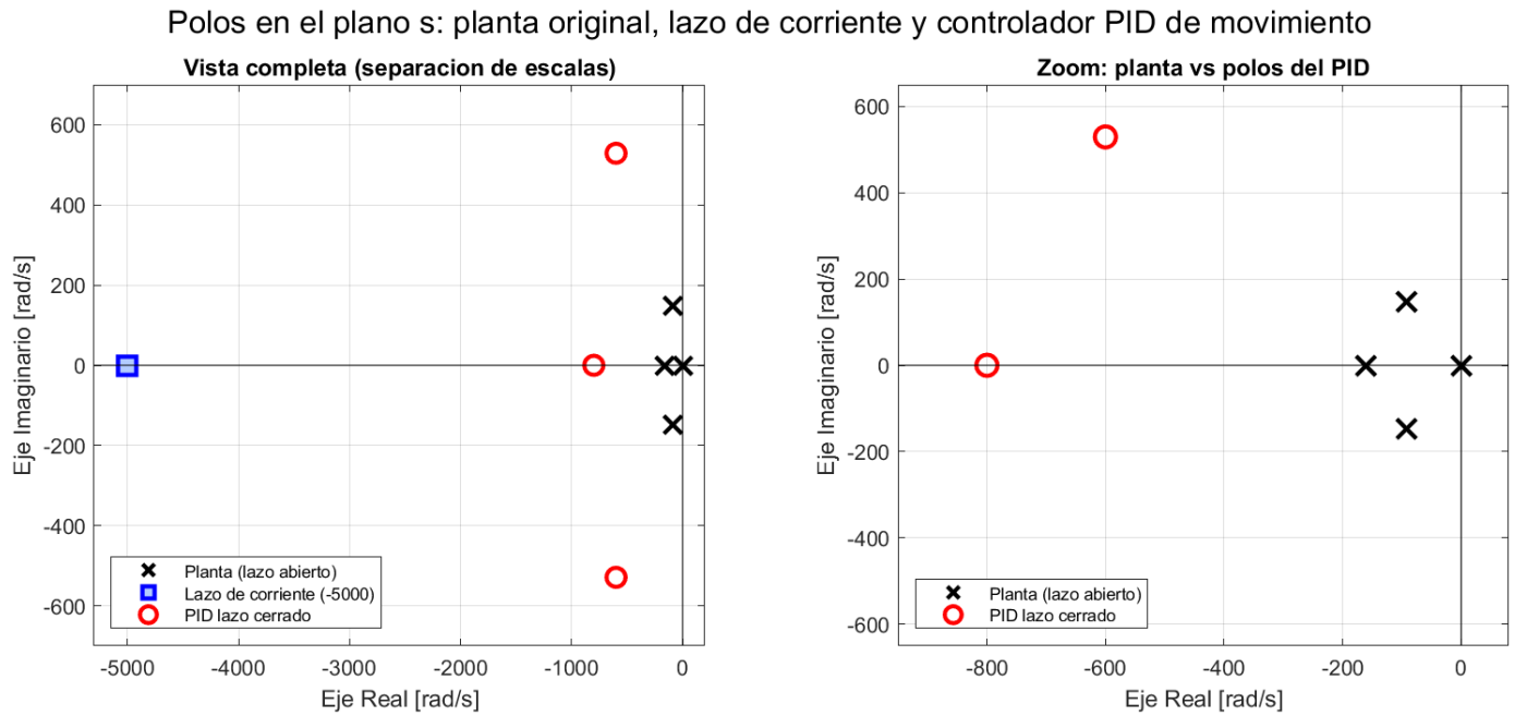
Fig. 39. Polos en el plano s : planta a lazo abierto (cruces), lazos de corriente (cuadrado, -5000 ) y polos de lazo cerrado del PID de movimiento (círculos, -800 y -600 \pm j529 ). Izquierda: vista completa (separación de escalas); derecha: zoom planta vs. PID.
