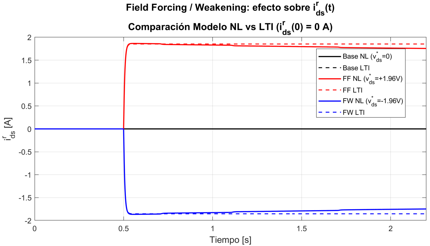
Fig. 30. Efecto del field forcing ( v_{ds}^{r*} = +1,96 V) y field weakening ( v_{ds}^{r*} = -1,96 V) sobre i_{ds}^r(t) , comparado con el caso base ( v_{ds}^{r*} = 0 ).
