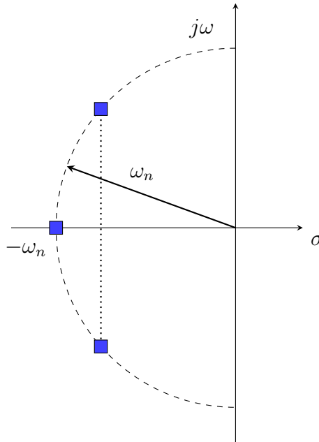
Fig. 38. Configuración de polos asignada por el polinomio requerido P_r(s) : polo real en -\omega_n y par complejo conjugado de parámetros \zeta y \omega_n . Los tres polos comparten la frecuencia natural \omega_n : yacen sobre la circunferencia punteada de radio \omega_n .
