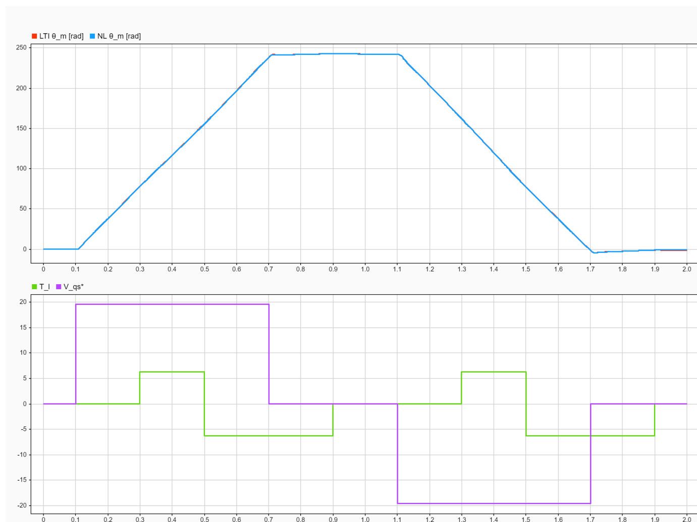
Fig. 16. Posición angular \theta_m(t) : comparación NL (azul) vs LTI aumentado (rojo). Panel inferior: señales de excitación (torque de carga T_i y consigna v_{qs}^{r*} ).
