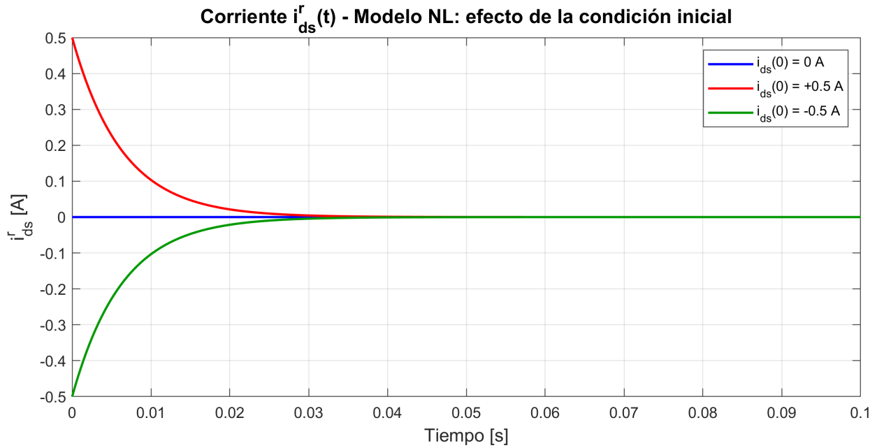
Fig. 27. Comparación de i_{ds}^r(t) para i_{ds}^r(0) \in \{0, +0,5, -0,5\} A: modelo NL.
