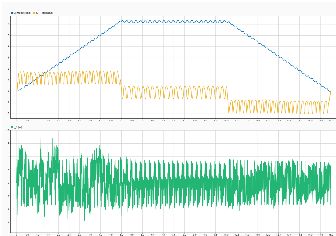
Fig. 57. Arriba: posición y velocidad; abajo: corriente en eje de cuadratura. Puede verse el efecto del modelo en SS de los sensores, con el cual el sistema no puede seguir la consigna de posición. ( T_{ld} = 5 [Nm])
