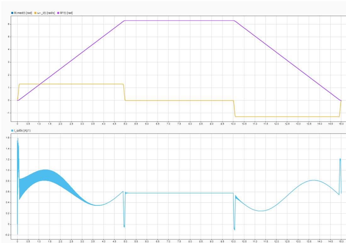
Fig. 60. Arriba: posición y velocidad; abajo: corriente en eje de cuadratura. Finalmente se consigue un desempeño satisfactorio y, al mismo tiempo, el cumplimiento de las demás condiciones de operación. ( T_{ld} = 5 [Nm], \omega_n = 12000 [rad/s])
