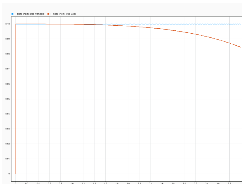
Fig. 33. Evolución temporal del torque neto ( T_{neto} ) en [N.m]. Se contrasta el comportamiento con resistencia estática constante (RS Cte., línea roja) y con resistencia estática variable (RS Variable, línea azul).
