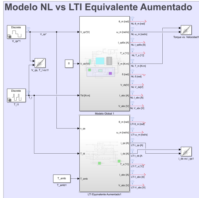
Fig. 15. Diagrama de bloques en Simulink: modelo NL desacoplado y LTI aumentado en paralelo frente a la misma consigna v_q^* y al mismo torque de perturbación.
