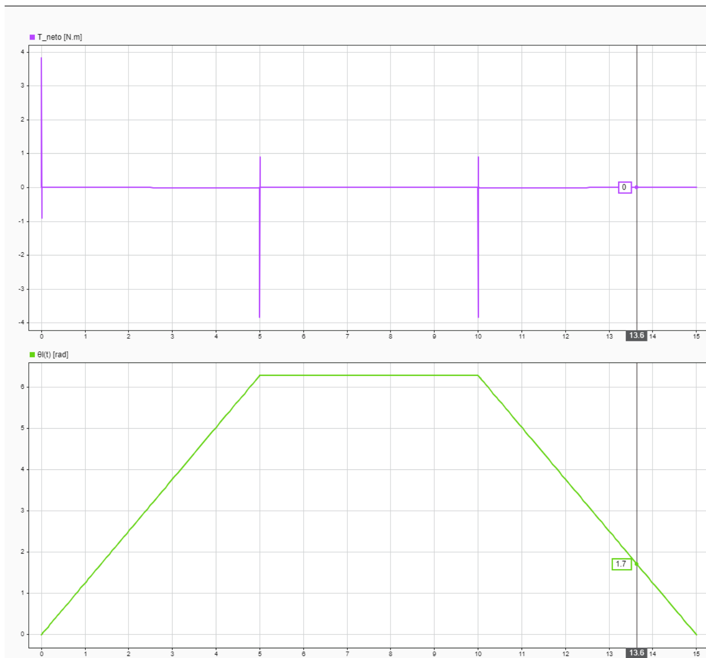
Fig. 43. Torque neto aplicado por la articulación para seguir la consigna de posición.
