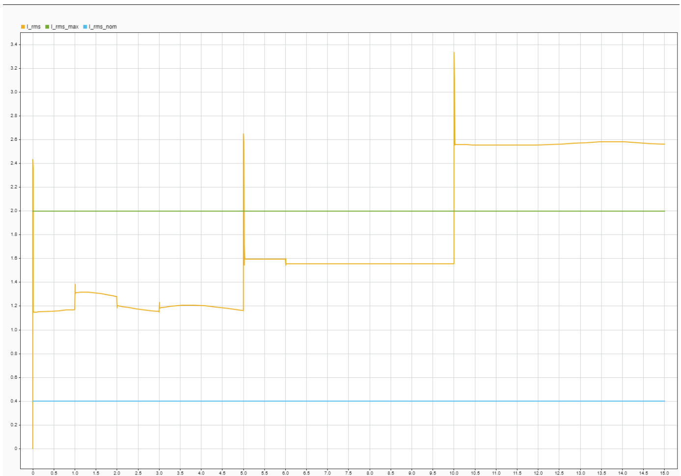
Fig. 50. Puede verse que, aun con saturación en la consigna de corriente, el accionamiento no puede cumplir la consigna sin superar sus especificaciones.
