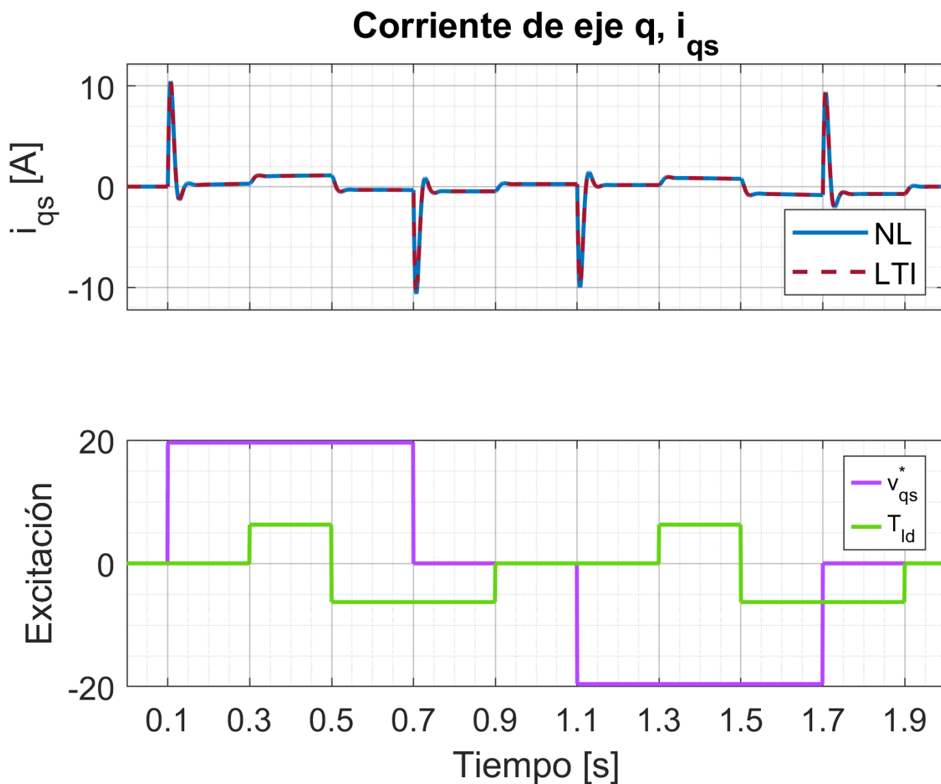
Fig. 20. Corriente de eje q, i_{qs}^r(t) : comparación NL (azul) vs LTI aumentado (rojo). Panel inferior: señales de excitación ( T_l y v_{qs}^{r*} ).
