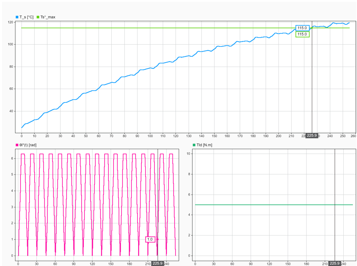
Fig. 58. Evolución de la temperatura del bobinado T_s(t) bajo operación repetitiva, considerando T_{amb}^{\circ} = 25^{\circ}\text{C} , T_{ld} = 5 \text{ Nm} y la consigna trapezoidal de posición utilizada en el trabajo. Se observa que la temperatura supera el límite admisible T_{s,max}^{\circ} = 115^{\circ}\text{C} a los 225.9 s.
