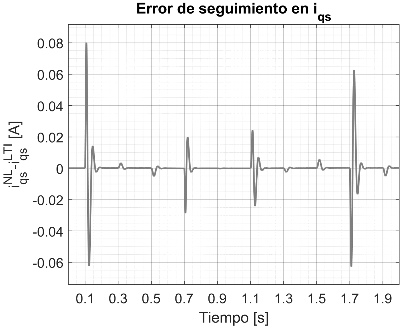
Fig. 21. Error de seguimiento en i_{qs}^r(t) : diferencia i_{qs}^{NL} - i_{qs}^{LTI} , nula en régimen y con picos \leq 0,1 A únicamente en las conmutaciones.
