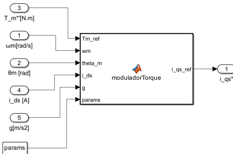
Fig. 67. Código implementado para el modulador de torque.
