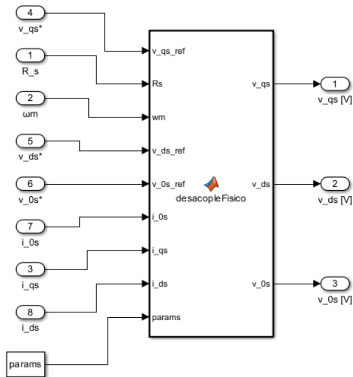
Fig. 69. Código implementado para el desacople de realimentaciones físicas naturales.
