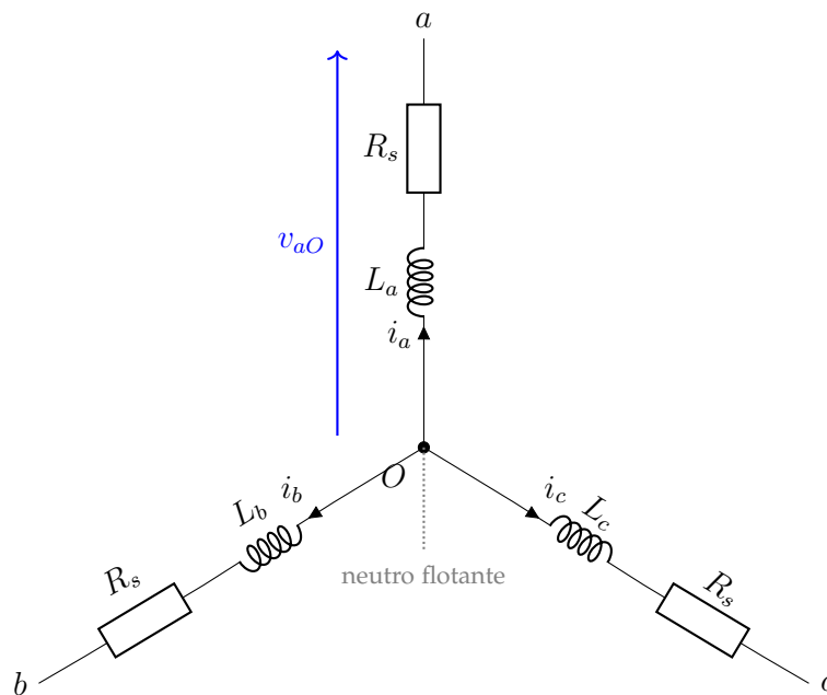
Fig. 2. Estator trifásico conectado en estrella con neutro flotante. Al no existir conductor de retorno externo, la Ley de Corrientes de Kirchhoff aplicada en el centro de estrella O impone i_a + i_b + i_c = 0 , por lo que la componente homopolar de corriente resulta nula: i_{0s}(t) \equiv 0 .
