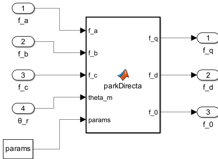
Fig. 70. Código implementado para la transformación directa de Park.
