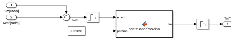
Fig. 65. Código implementado para el controlador PID de posición.
