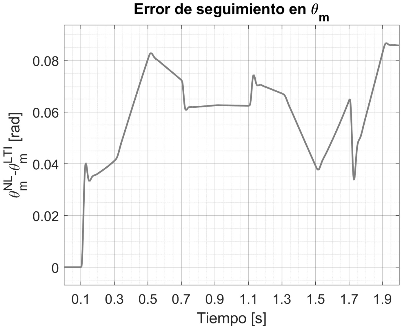
Fig. 17. Error de seguimiento en \theta_m(t) : diferencia \theta_m^{NL} - \theta_m^{LTI} , acotada por debajo de 0,1 rad ( < 0,05\% de la excursión de 242 rad).
