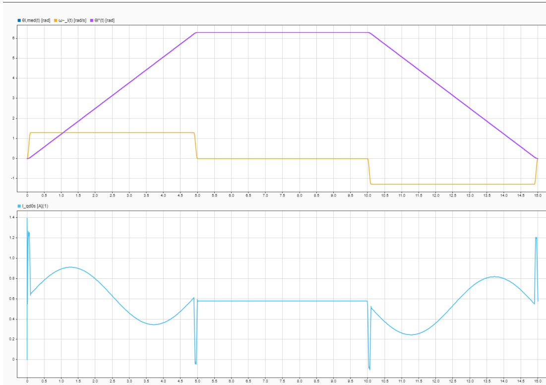
Fig. 60. Arriba: posición y velocidad; abajo: corriente en eje de cuadratura. Puede verse que el accionamiento ya sigue con éxito la consigna solicitada, sin oscilaciones producidas por los retardos de los sensores. ( T_{ld} = 5 [Nm])
