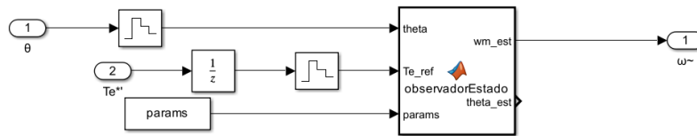
Fig. 66. Código implementado para el observador de estado de velocidad.
