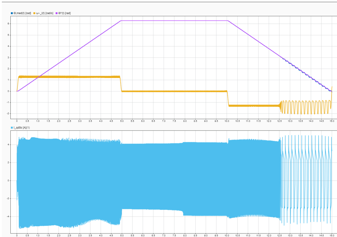
Fig. 61. Arriba: posición y velocidad; abajo: corriente en eje de cuadratura. Puede verse que el inversor no es lo suficientemente rápido. ( T_{ld} = 5 [Nm], \omega_n = 6000 [rad/s])
