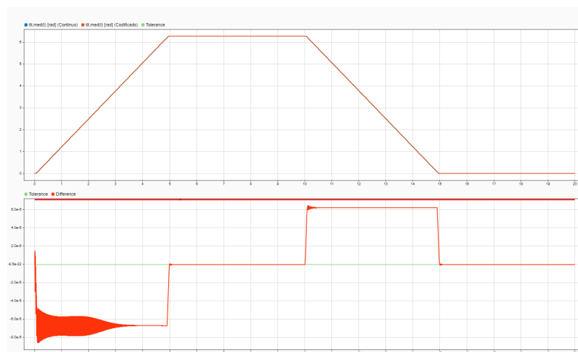
Fig. 72. Comparación de seguimiento de consigna de posición del modelo continuo vs el codificado discreto.
