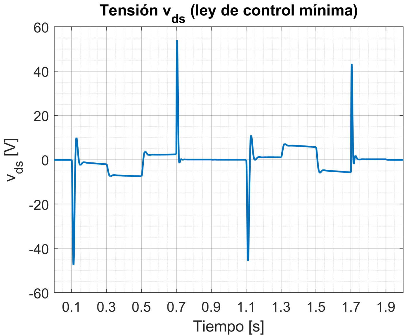
Fig. 23. Tensión v_{ds} vs t : modelo NL ( i_{ds}^r(0) = 0 A).
