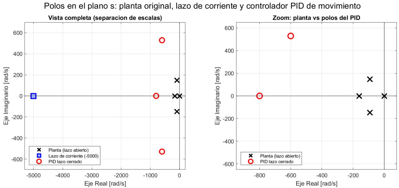
Fig. 40. Polos en el plano s : planta a lazo abierto (cruces), lazos de corriente (cuadrado, -5000 ) y polos de lazo cerrado del PID de movimiento (círculos, -800 y -600 \pm j529 ). Izquierda: vista completa (separación de escalas); derecha: zoom planta vs. PID.
