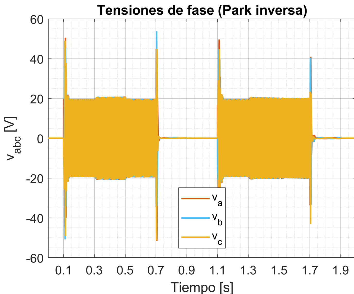
Fig. 25. Tensiones de fase v_a , v_b , v_c aplicadas al estator (modelo NL, i_{ds}^r(0) = 0 A), con el mismo código de colores por fase que las corrientes.
