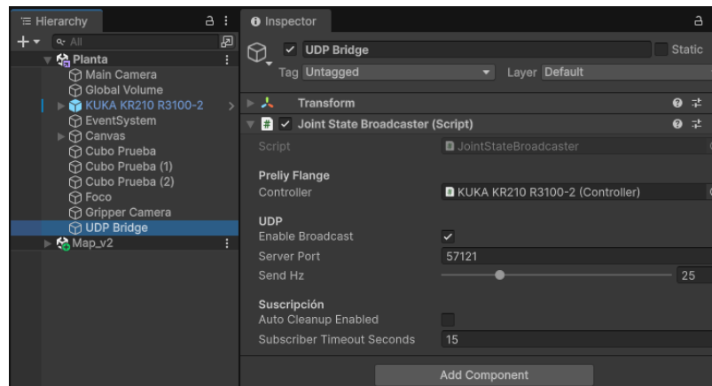
Figura 44: GameObject UDP Bridge: componente JointStateBroadcaster con el Controller de Preliy Flange, puerto, frecuencia de envío y parámetros de suscripción.
