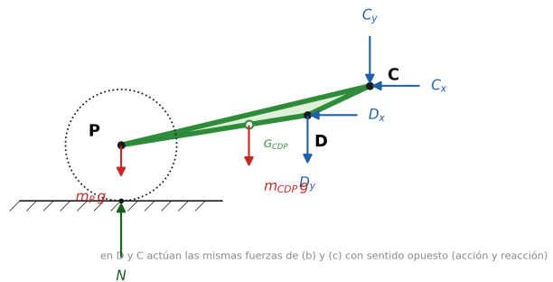
(d) Acoplador CDP con rueda y motor
