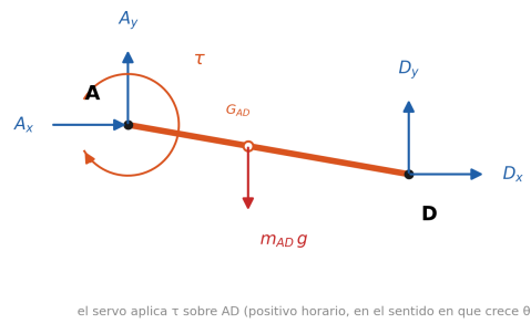
(b) Manivela AD
