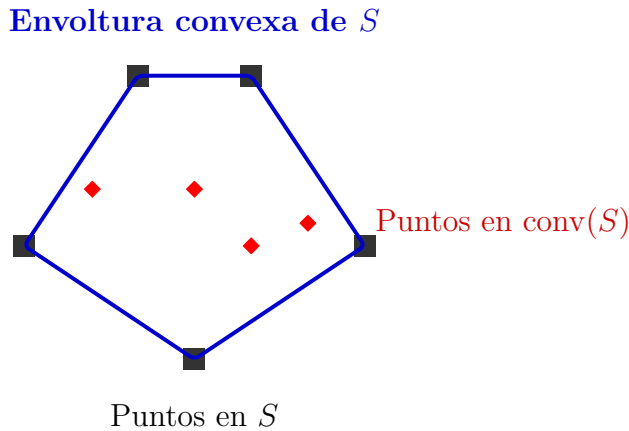
Figura A.1: Visualización de la envoltura convexa de un conjunto de puntos en \mathbb{R}^2 .
