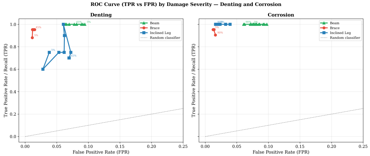
Figure 16: Curvas ROC para el clasificador de daño mediante ICD: Abolladura (izq.) y Corrosión (der.). Valores resumen: AUC-ROC (Abolladura) > 0.90; AUC-ROC (Corrosión) > 0.94. Punto operativo sugerido: si se prioriza baja tasa de falsas alarmas seleccione el umbral cercano al marcador 'Brace (5%)' (TPR \approx 0.90, FPR \approx 0.01).
