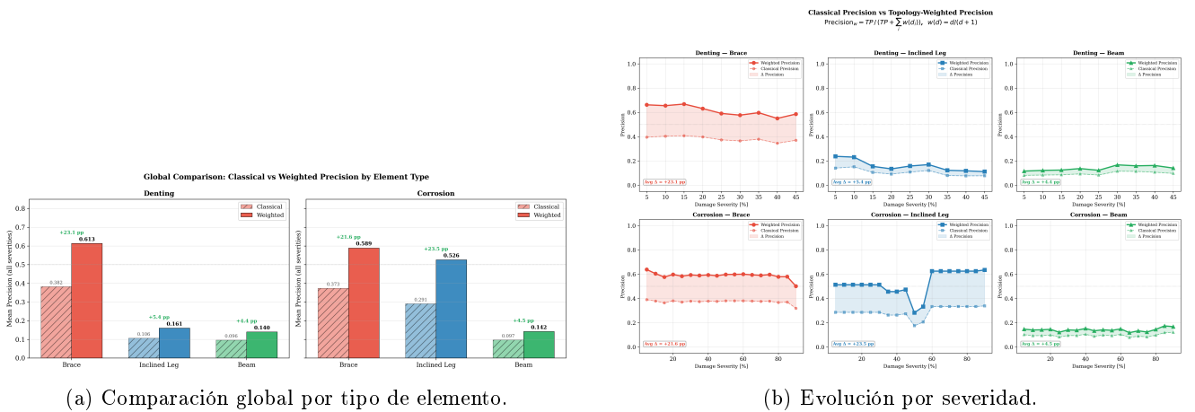
Figure 20: (a) Comparación global de Precision Clásica vs. Ponderada por tipo de elemento; (b) Evolución de la Precision Clásica (línea punteada) y Ponderada (línea sólida) en función de la severidad del daño. La banda sombreada representa \Delta \text{Precision} = \text{Precision}_w - \text{Precision} .
