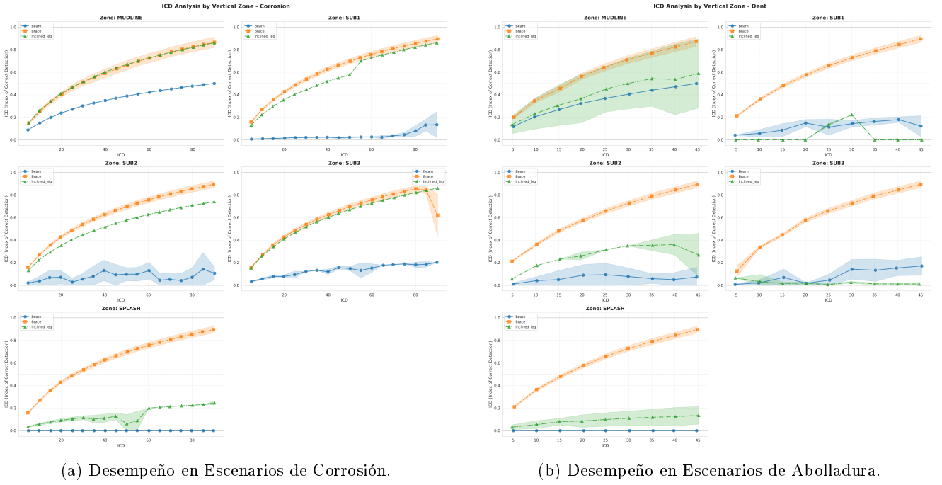
Figure 12: Influencia de la ubicación vertical del daño en la calidad de detección (ICD).
