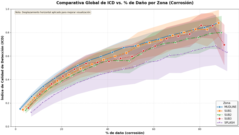
Figura: Comparativa Global ICD vs Severidad de Daño (Corrosión)
