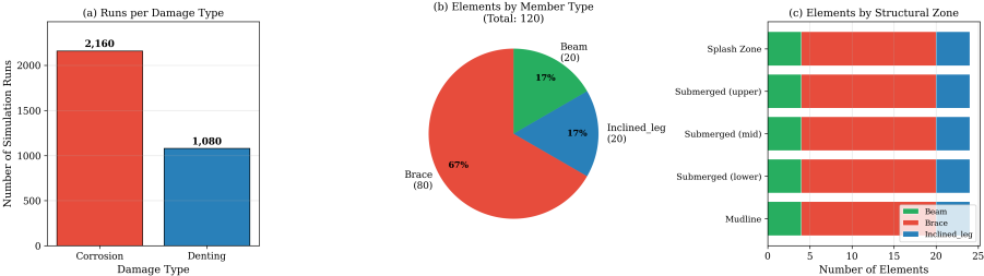
Figura: Distribución del diseño experimental: elementos y niveles de severidad
