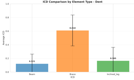
Figure 8: Comparativa de sensibilidad del ICD por tipo de elemento bajo escenarios de abolladura.
