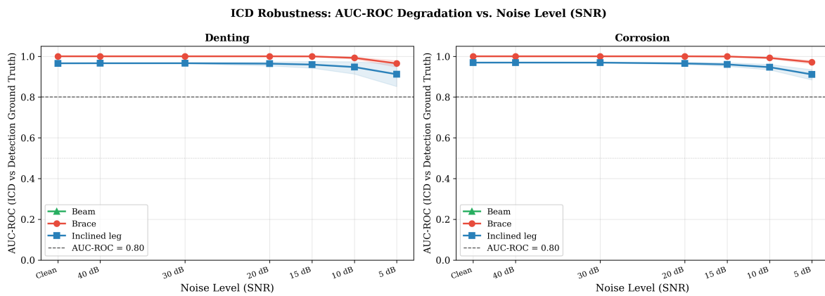
Figure 12: Degradación del AUC-ROC en función del nivel de ruido (SNR) para Abolladura (izq.) y Corrosión (der.). Línea punteada = umbral de AUC = 0.80.
