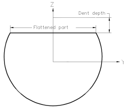
Figure 1: Parametrización de la sección transversal abollada.
