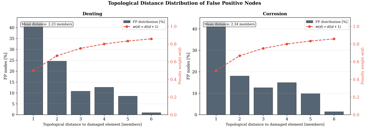
Figure 14: Distribución de distancias topológicas de los nodos FP al elemento dañado para Abolladura (izq.) y Corrosión (der.). La curva roja muestra la función de peso w(d) = d/(d+1) .
