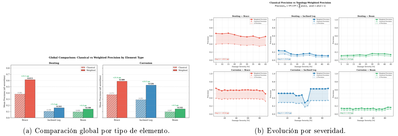
Figure 15: (a) Comparación global de Precision Clásica vs. Ponderada por tipo de elemento; (b) Evolución de la Precision Clásica (línea punteada) y Ponderada (línea sólida) en función de la severidad del daño. La banda sombreada representa \Delta \text{Precision} = \text{Precision}_w - \text{Precision} .
