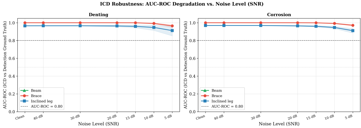
Figure 13: Degradación del AUC-ROC en función del nivel de ruido (SNR) para Abolladura (izq.) y Corrosión (der.). Línea punteada = umbral de AUC = 0.80.
