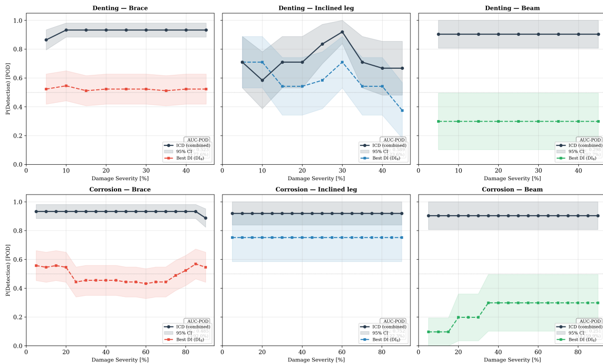
Figure 12: Curvas POD del ICD frente al mejor DI individual por tipo de elemento. Abolladura (fila superior) y Corrosión (fila inferior).
