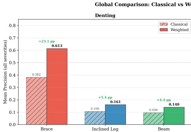
Figure 19: Comparación global de Precision Clásica vs. Ponderada por tipo de elemento. Las anotaciones indican el incremento \Delta en puntos porcentuales.
