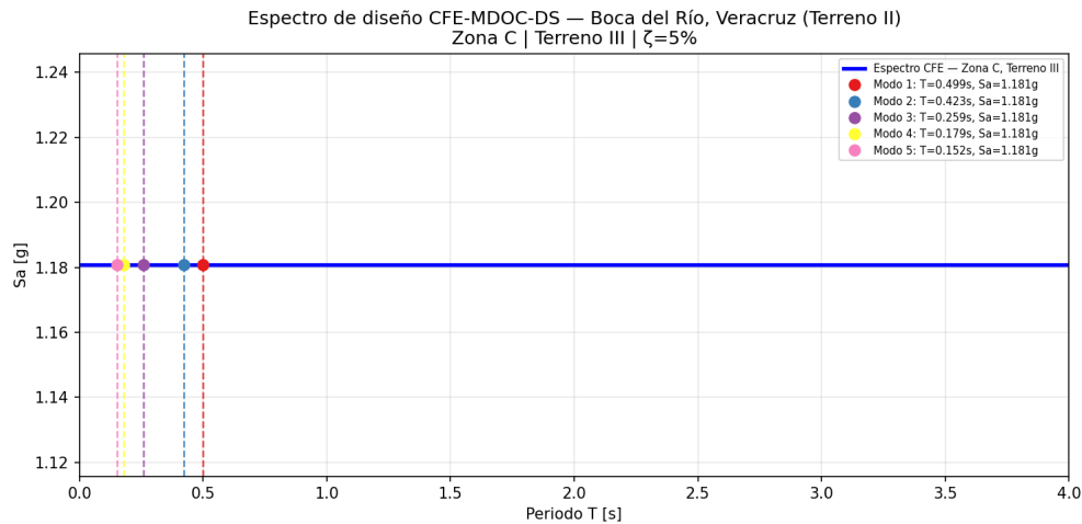
Figura 4: Espectro de diseño CFE C.1.3 — Zona C, Terreno III. Punto T_1 = 0.499 s marcado.
