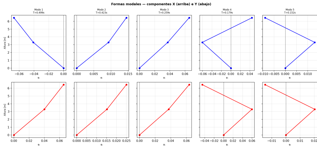
Figura 3: Primeras formas modales de vibración.
