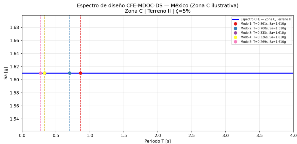
Figura 4: Espectro de diseño CFE C.1.3 — Zona C, Terreno II. Punto T_1 = 0.861 s marcado.
