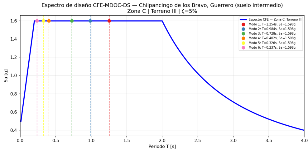
Figura 4: Espectro de diseño CFE C.1.3 — Zona C, Terreno III. Punto T_1 = 1.254 s marcado.
