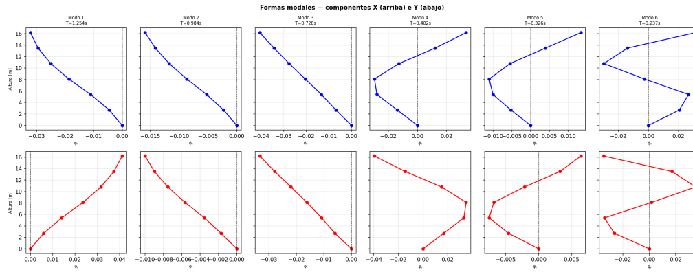
Figura 3: Primeras formas modales de vibración.
