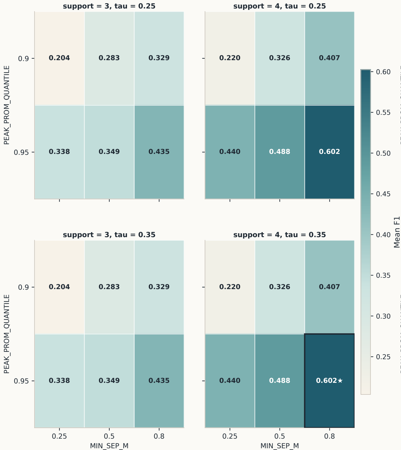
(a) Synthetic mean F1
