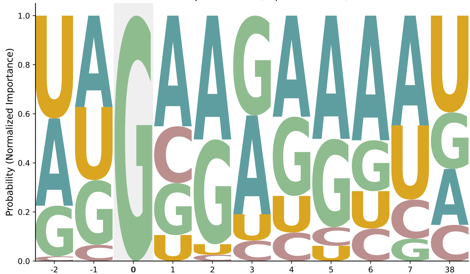
m7G: Spatial Motif (Top 10 Context)
