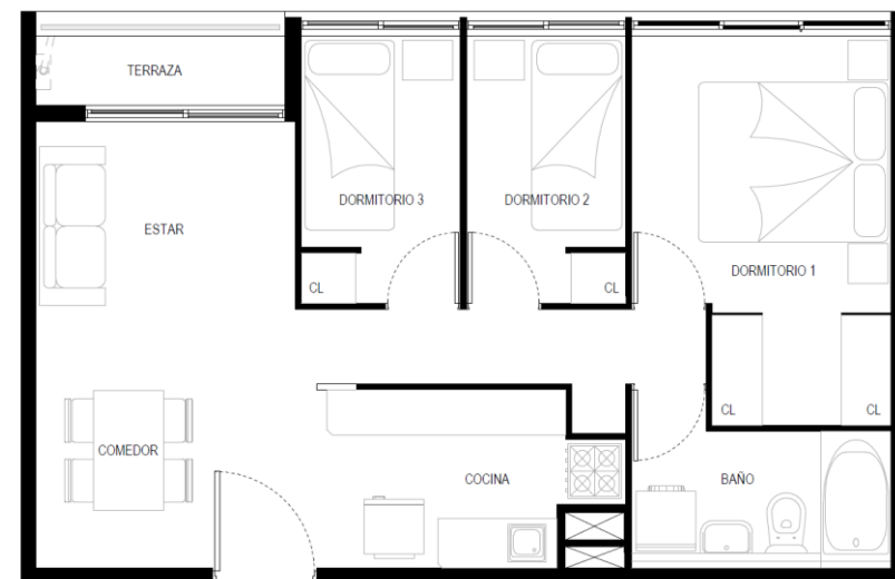
TIPOLOGÍA 3D1B (19 UNIDADES)
