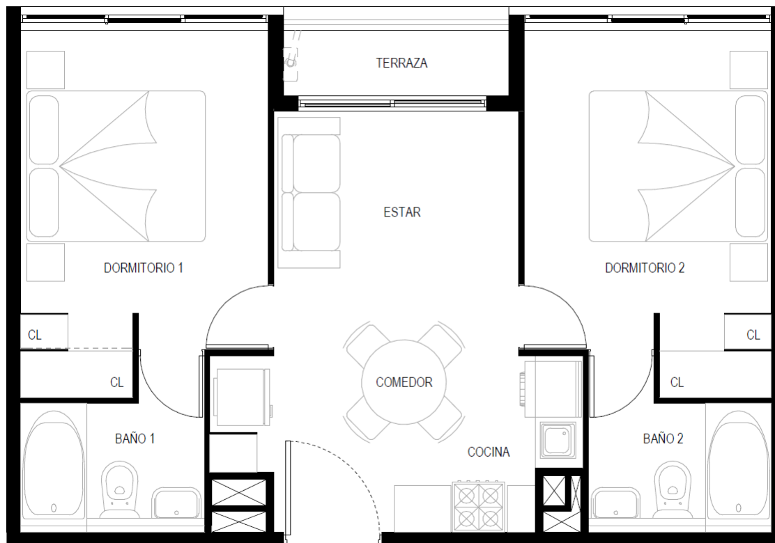
TIPOLOGÍA 2DBM (28 UNIDADES)
