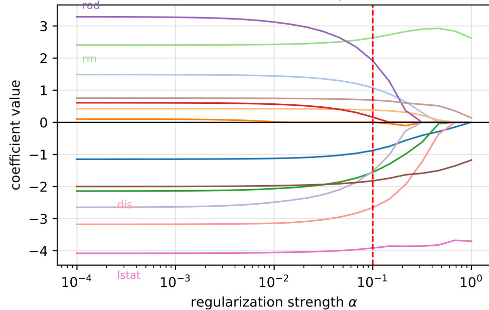
(d) Lasso: coefficient paths
