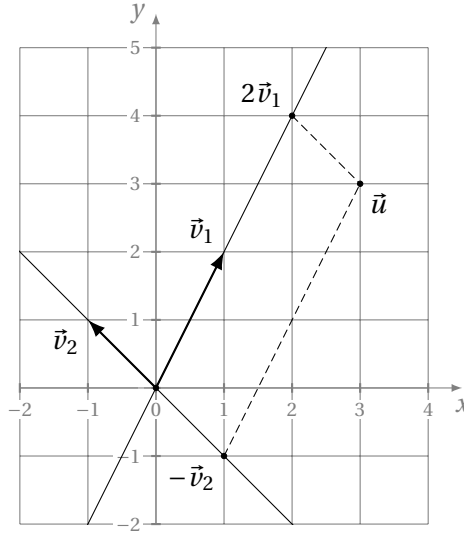
Figure 4.8 – Vecteurs de l'exemple 4.5.13.
