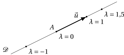
Figure 4.5 – Droite paramétrée.
