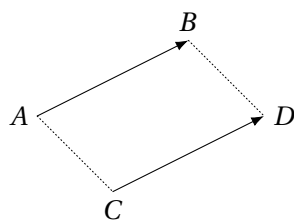
Figure 4.1 – Segments orientés équipollents.
