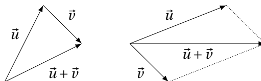
Figure 4.2 – Relation de Chasles et règle du parallélogramme.
