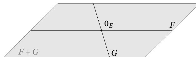
Figure 4.9 – Somme de sous-espaces vectoriels.
