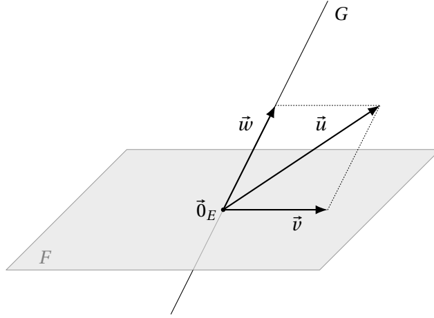
Figure 4.10 – Un plan et une droite supplémentaires dans \mathbb{R}^3 . Tout vecteur \vec{u} de \mathbb{R}^3 se décompose de manière unique comme la somme d'un vecteur du plan F et d'un vecteur de la droite G .
