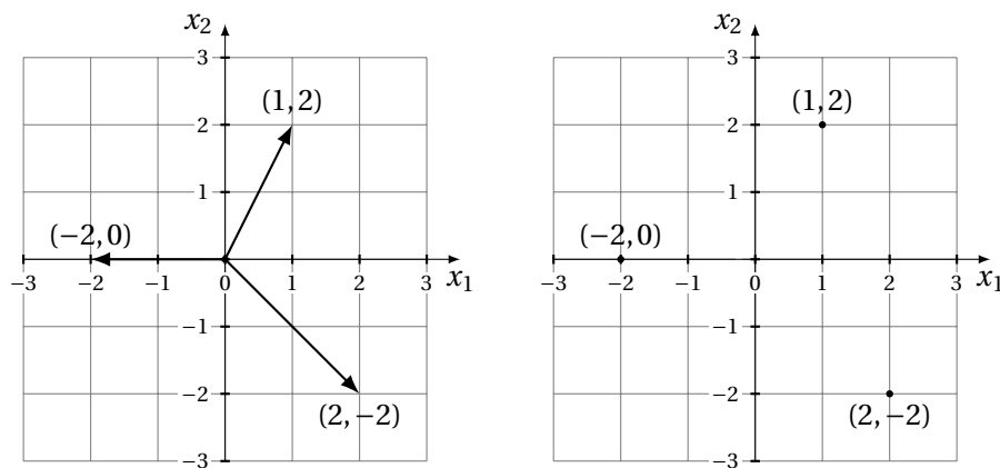
Figure 4.6 – Représentation des éléments de \mathbb{R}^2 comme des segments orientés ou comme des points.
