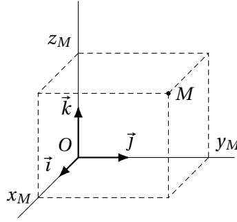
Figure 4.4 – Coordonnées d'un point dans un repère de l'espace.
