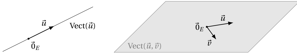
Figure 4.7 – Droite vectorielle et plan vectoriel.
