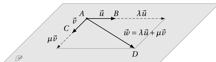
Figure 4.3 – Vecteurs coplanaires.
