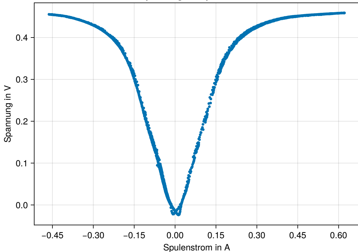
Spannung vs. Spulenstrom
