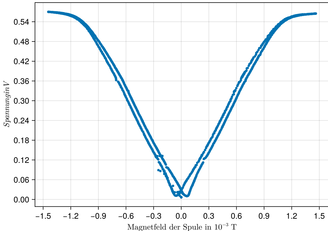
Eichkurve von Sensor 1
