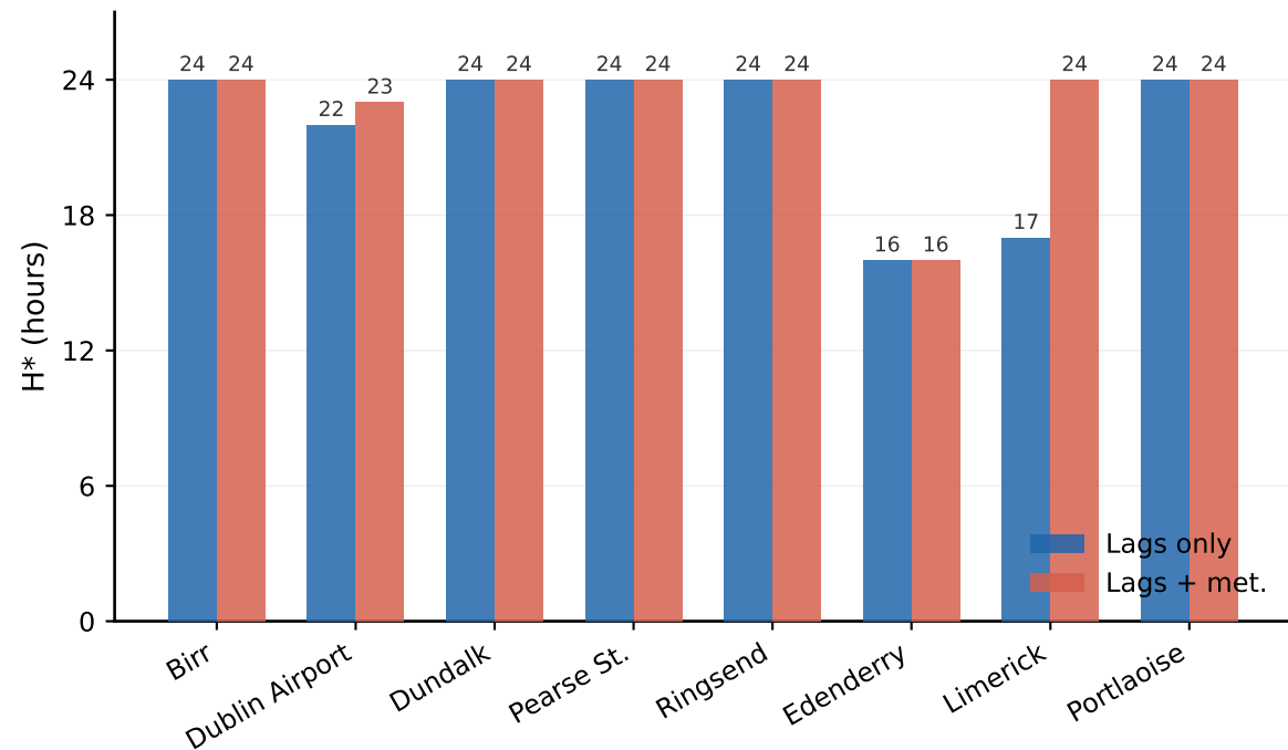
H* strict (max-run)
