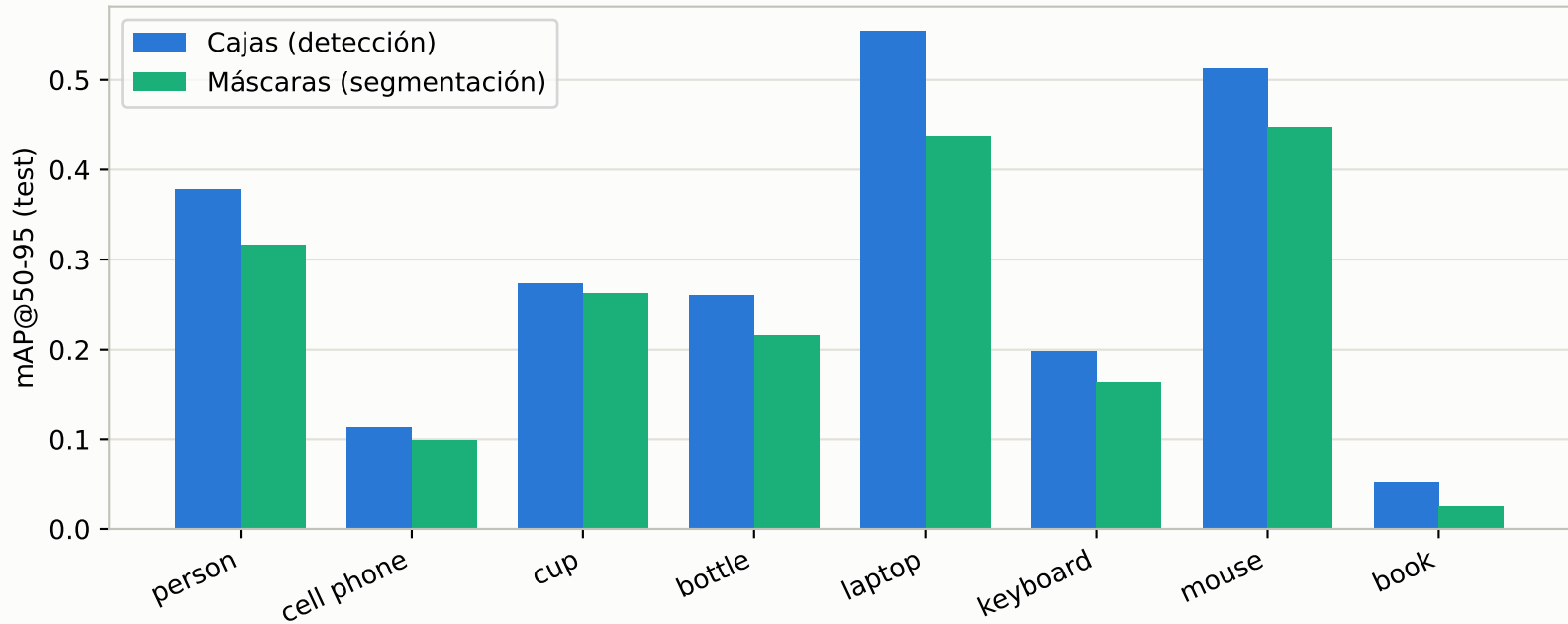
Desempeño por clase sobre la partición de prueba
