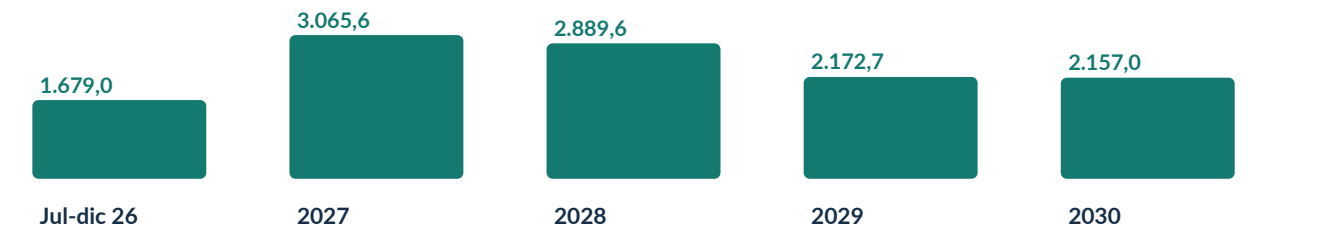
Pagos previstos: capital + intereses
