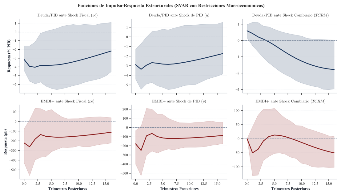
Figura 8: Funciones de Impulso-Respuesta Estructurales (SVAR Restringido) con Bandas Bootstrap al 95 %.
