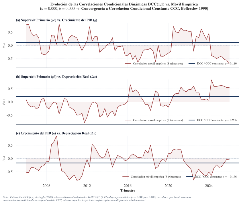
Figura 6: Evolución Temporal de las Correlaciones Dinámicas Condicionales (DCC-GARCH).
