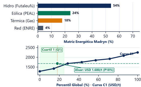
Figura 10: Matriz Renovable y Curva C1: Posicionamiento en el primer cuartil de costos de fundición.
