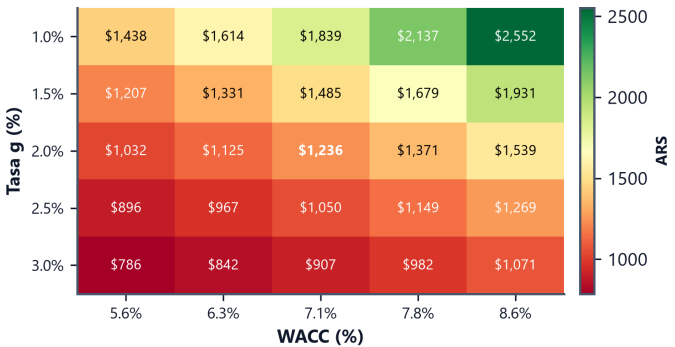
Figura 13: Matriz de sensibilidad bidimensional del Precio Objetivo (ARS) ante variaciones en WACC y tasa de crecimiento perpetuo g .
