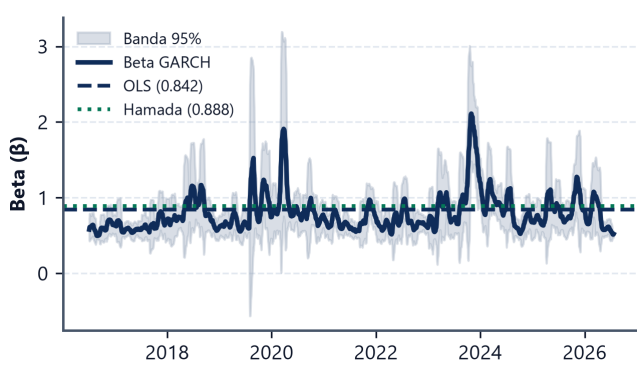
Figura 30: Beta Condicional GARCH(1,1): Variación temporal de la volatilidad y riesgo sistemático.
