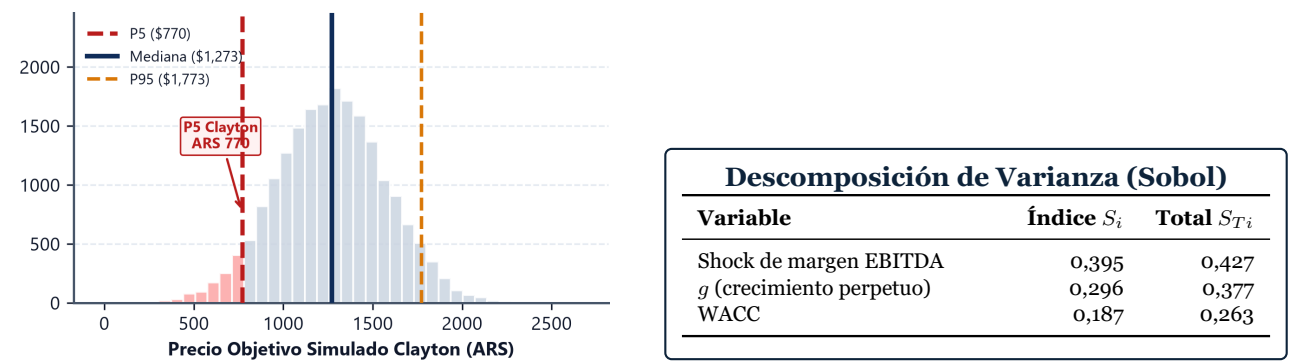
Figura 31: Ajuste de Cópula de Clayton: Ilustra la dependencia de cola inferior ( \lambda_L = 0,53 ). El ajuste por AIC favorece finalmente a la t -Student (cola simétrica, ver texto).
