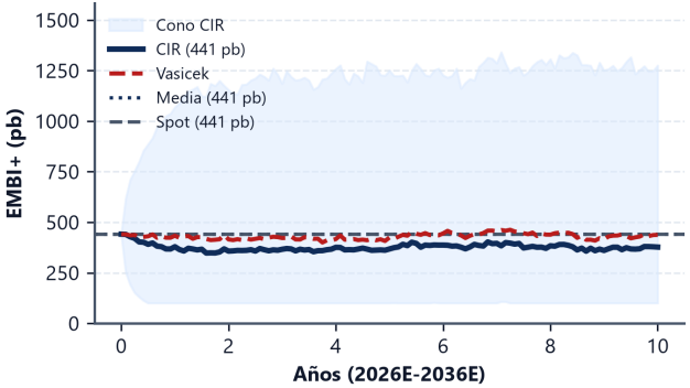
Figura 28: Proceso CIR Soberano: Simulación condicional anclada a 441 pb con no-negatividad estricta.
