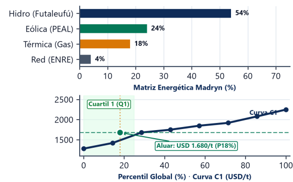
Figura 10: Matriz Renovable y Curva C1: Curva global de costos y posición de Aluar.
