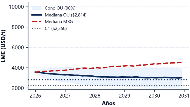
Figura 27: Simulación LME (OU vs. MBG): Reversión a la media Ornstein-Uhlenbeck ( \theta = USD 2.814/t).
