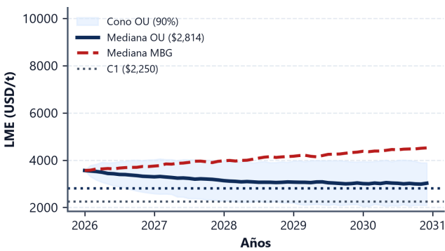
Figura 26: Simulación LME (OU vs. MBG): Reversión a la media Ornstein-Uhlenbeck ( \theta = \text{USD } 2.814/\text{t} ).
