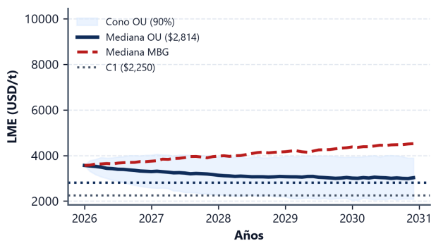
Figura 25: Proceso Ornstein-Uhlenbeck LME (Cono 90 %) vs MBG.
