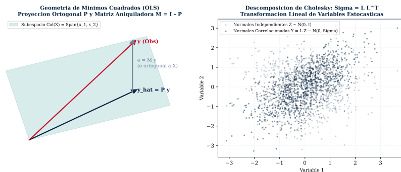
Figura 15: Figura Teórica: Geometría de Hilbert de Proyecciones OLS y Factorización de Cholesky \Sigma = \mathbf{L}\mathbf{L}^T .
