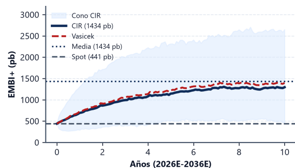
Figura 21: Difusión CIR vs Vasicek para curva de tasas y EMBI+.
