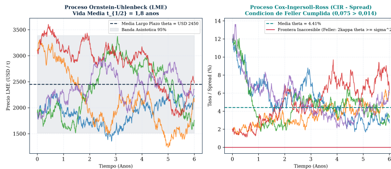
Figura 19: Figura Teórica: Trayectorias Estocásticas de Ornstein-Uhlenbeck (LME) y Proceso CIR con Condición de Feller.
