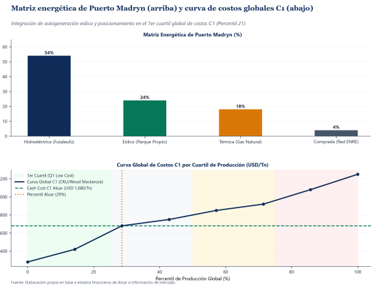
Figura 10: Matriz energética de Puerto Madryn (arriba) y curva de costos globales C1 (abajo).
