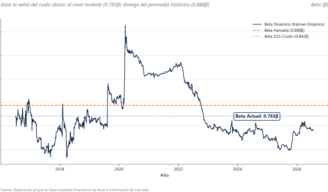
Figura 24: Trayectoria estocástica del Beta Dinámico estimado por Filtro de Kalman (2016-2026): identifica el régimen de riesgo más reciente del activo.
