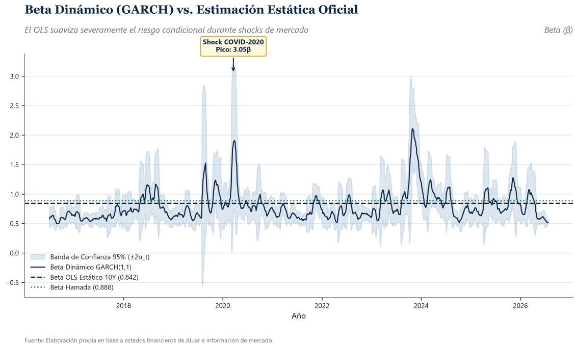
Figura 30: Beta Dinámico (GARCH) vs. Estimación Estática Oficial. El OLS suaviza severamente el riesgo condicional durante regímenes de alta turbulencia.
