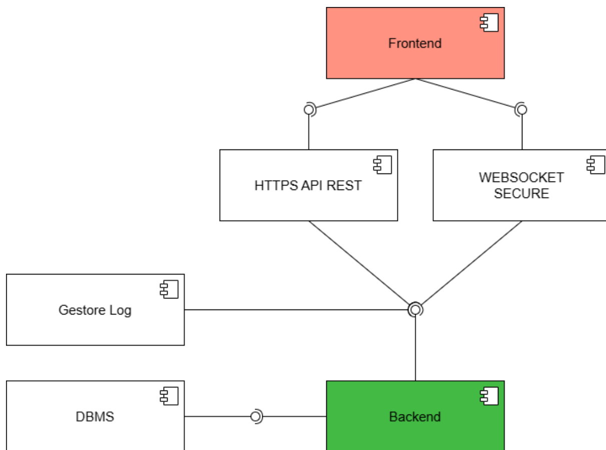
Figura 3.2: Diagramma dei componenti
