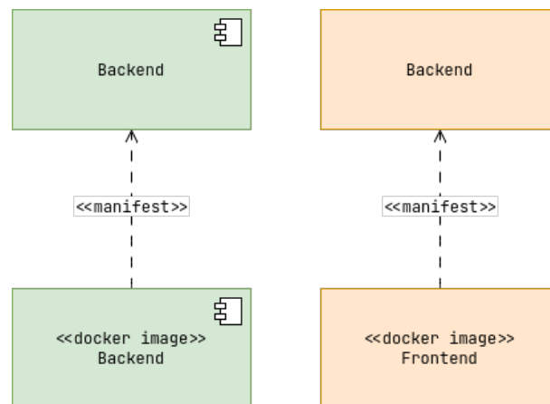
Figura 3.9: Diagramma degli artefatti
